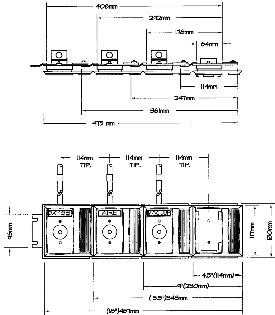
DT-16 CAJA DE VALVULA - INCRUSTADO (TIPICO) GM-4 SIN ESCALA
