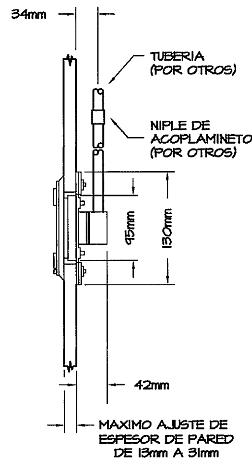
DT-18 SALIDA DE GASES DE PARED "SGM" (TIPICO) GM-4 SIN ESCALA
