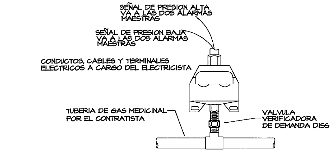
DT-20 SENSOR DE PRESION ALTA / BAJA (TIPICO) GM-4 SIN ESCALA
