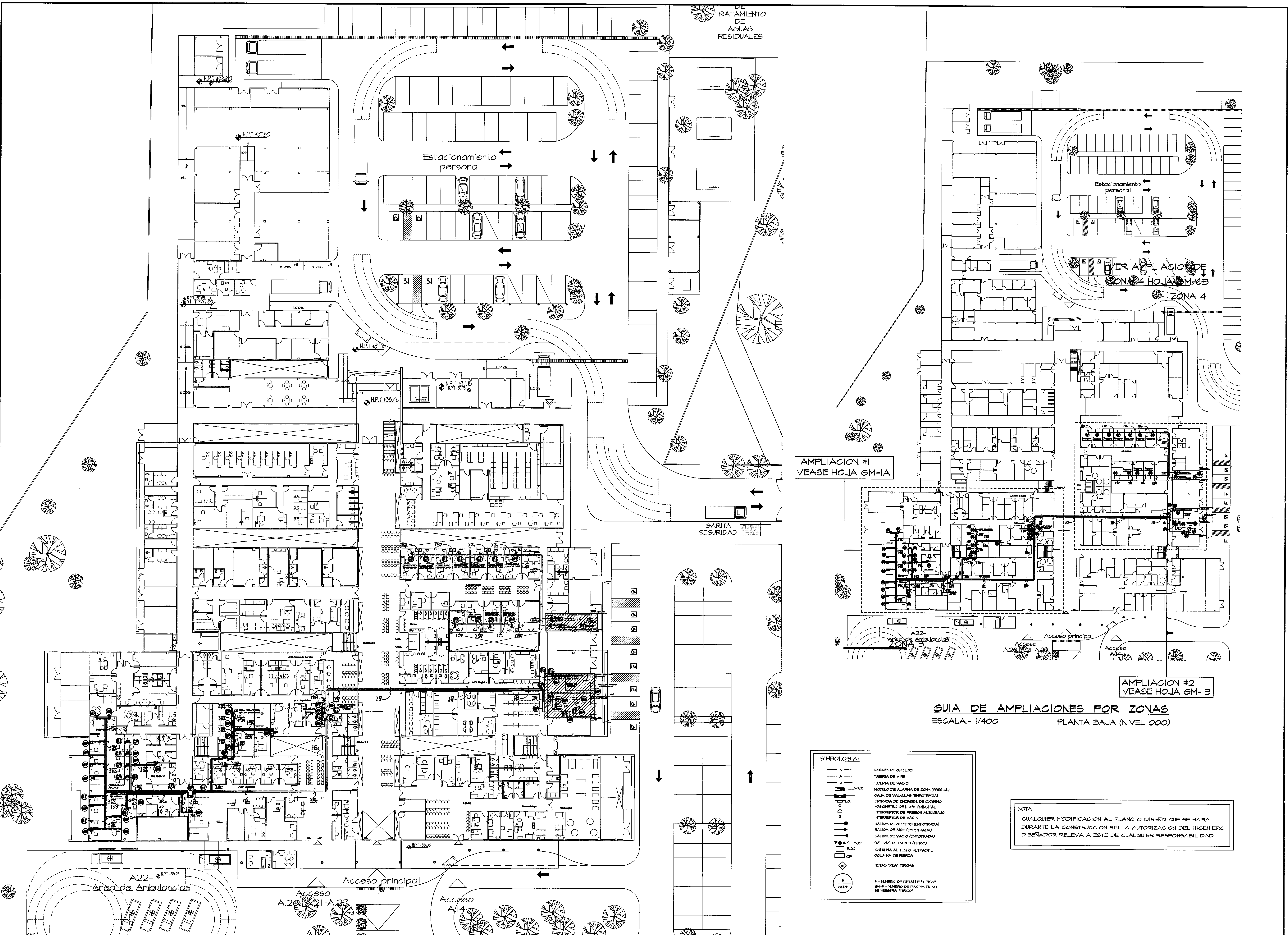
PLANTA DE GASES MEDICOS-RECORRIDO GENERAL- PLANTA BAJA ESCALA 1:250
