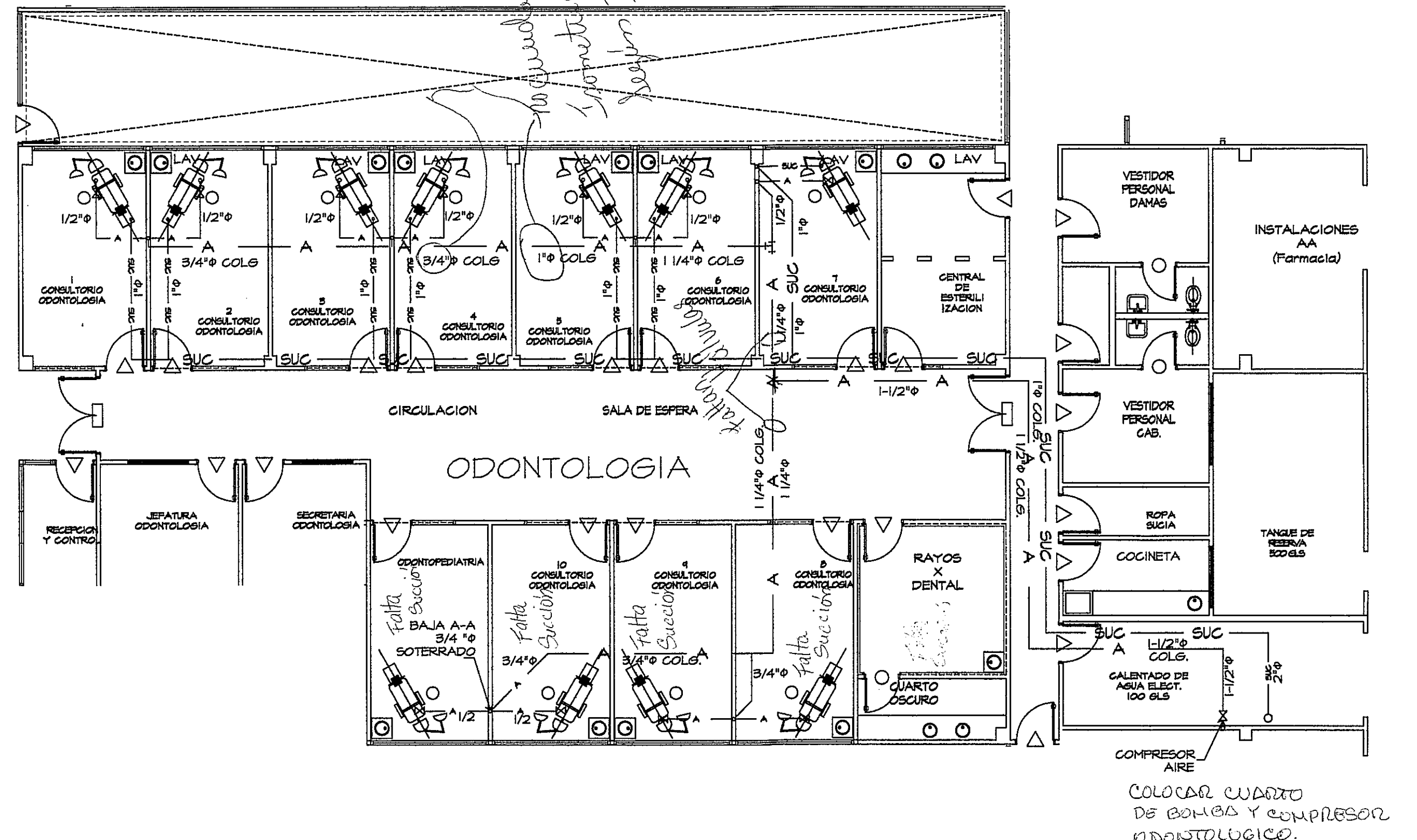
PLANTA AMPLIACION ZONA 4 SISTEMA AIRE Y SUCCION NIVEL 000
