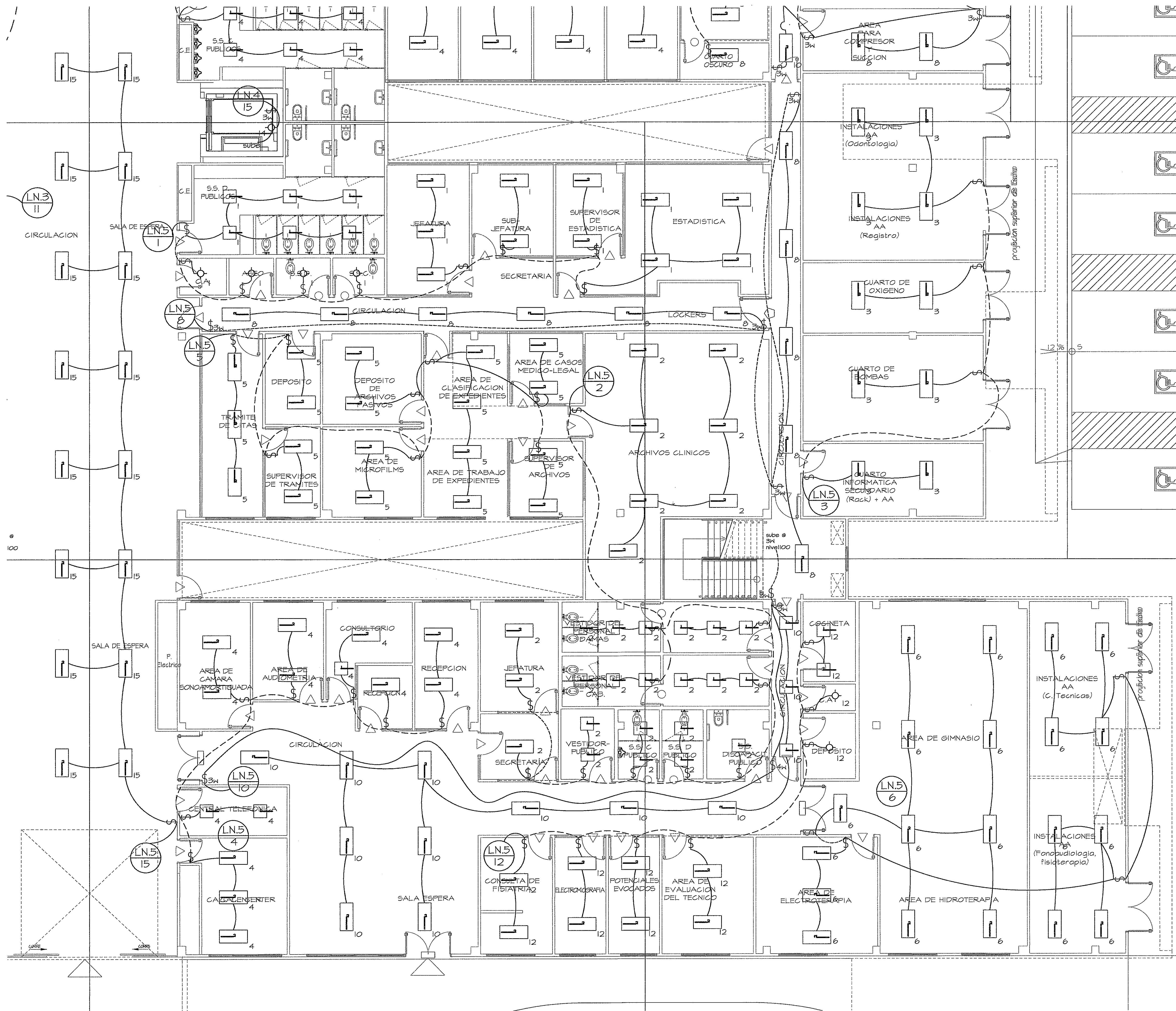
AMPLIACION DE ZONA 5 ESCALA 1:75 PLANTA BAJA
