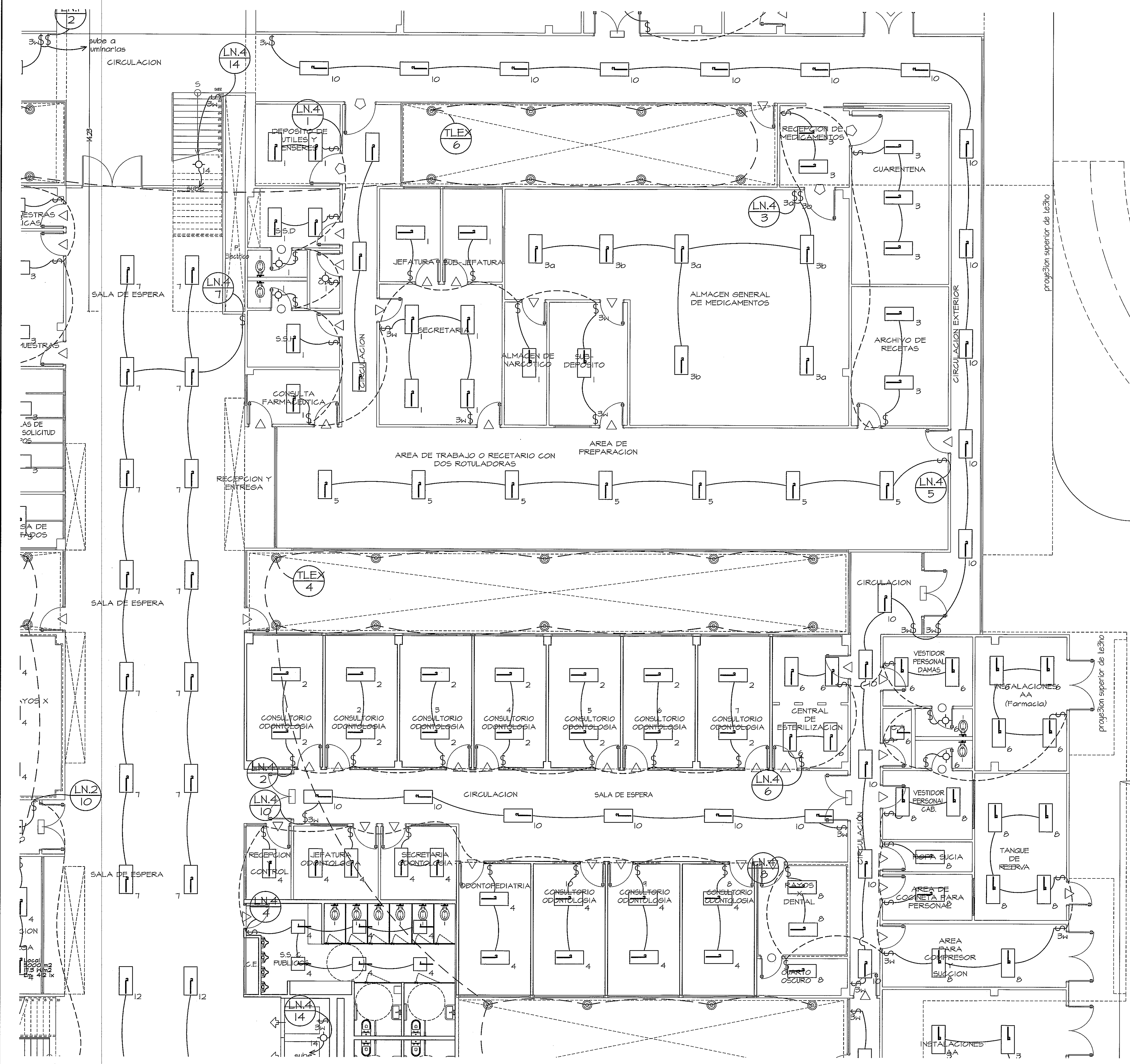
AMPLIACION DE ZONA 4 ESCALA 1:75 PLANTA BAJA
