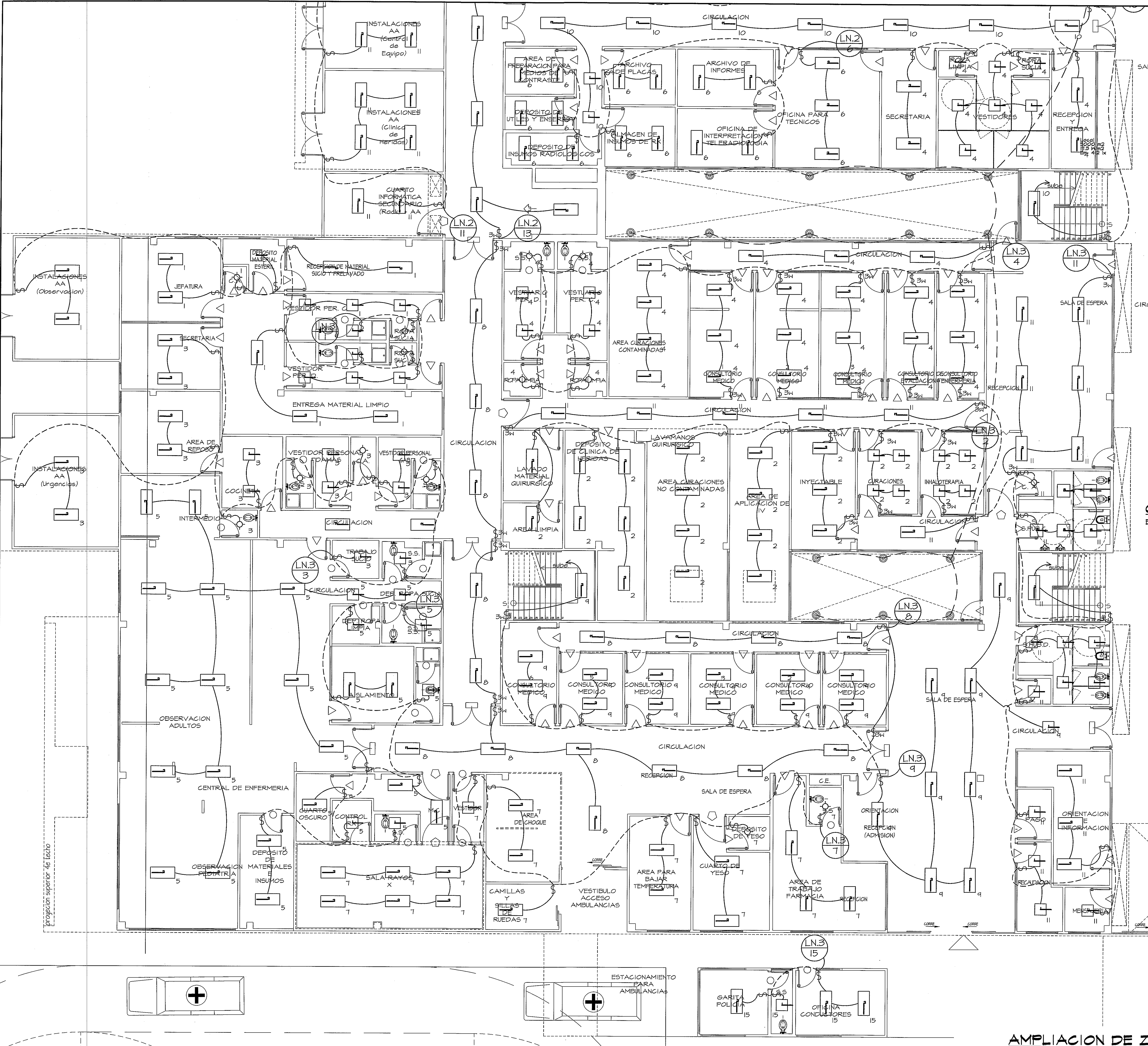
ZONA 3 GUÍA DE AMPLIACIONES POR SECCIÓN ESCALA 1:650 PLANTA BAJA (NIVEL 000)
