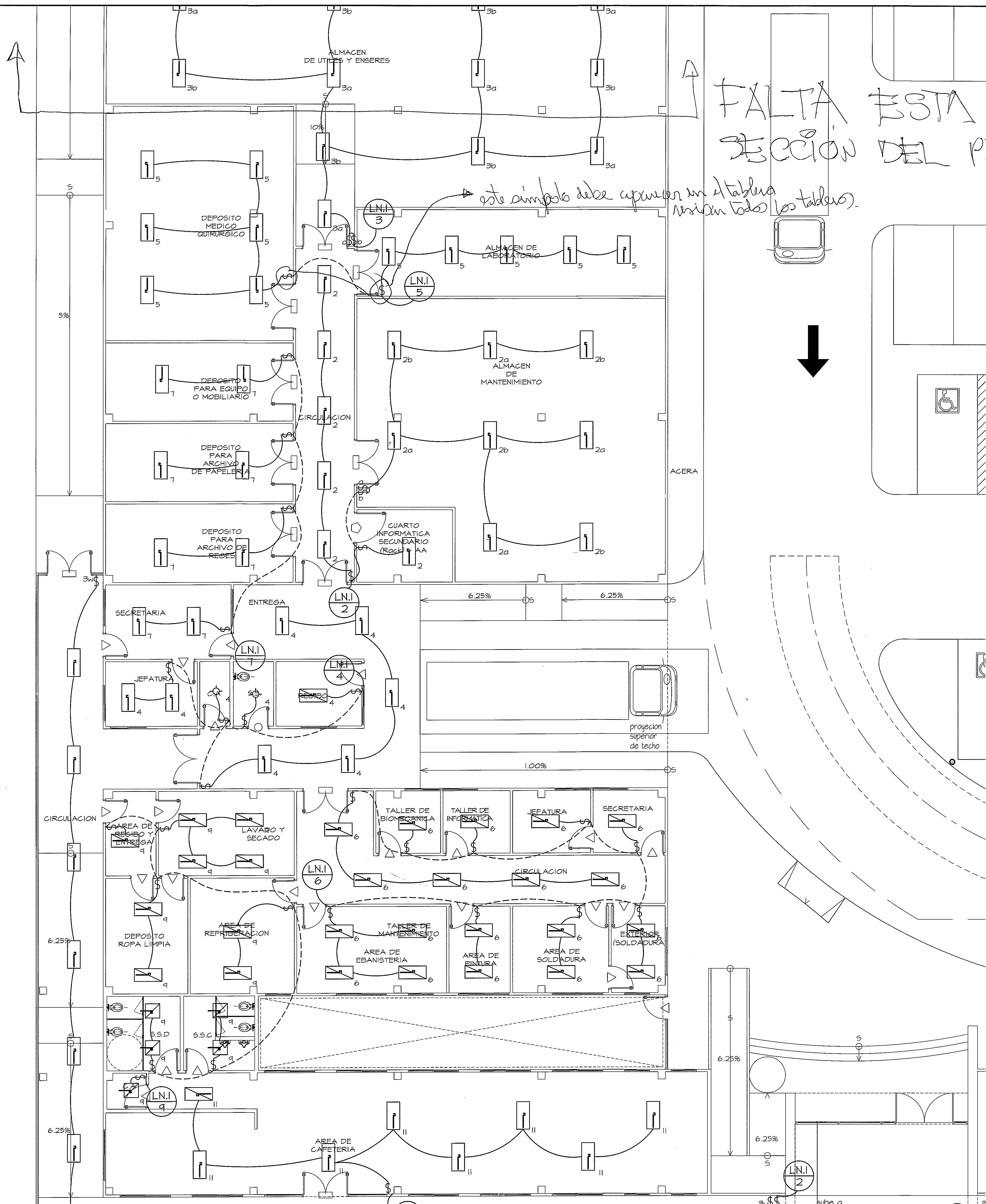
AMPLIACION DE ZONA I ESCALA 1:75 PLANTA BAJA
