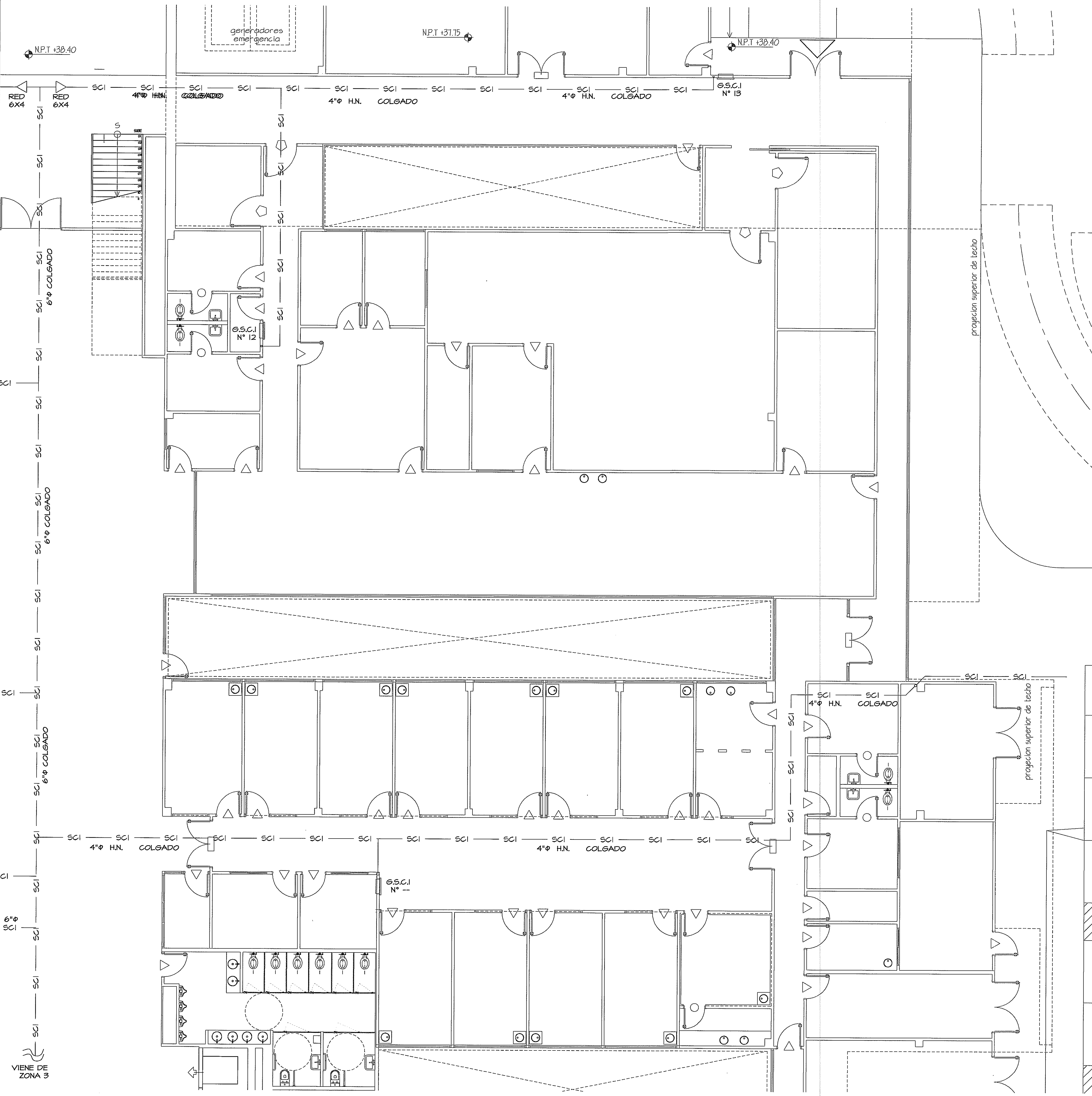
PLANTA AMPLIACION DE ZONA 4 SISTEMA CONTRA INCENDIO ESCALA 1:75
