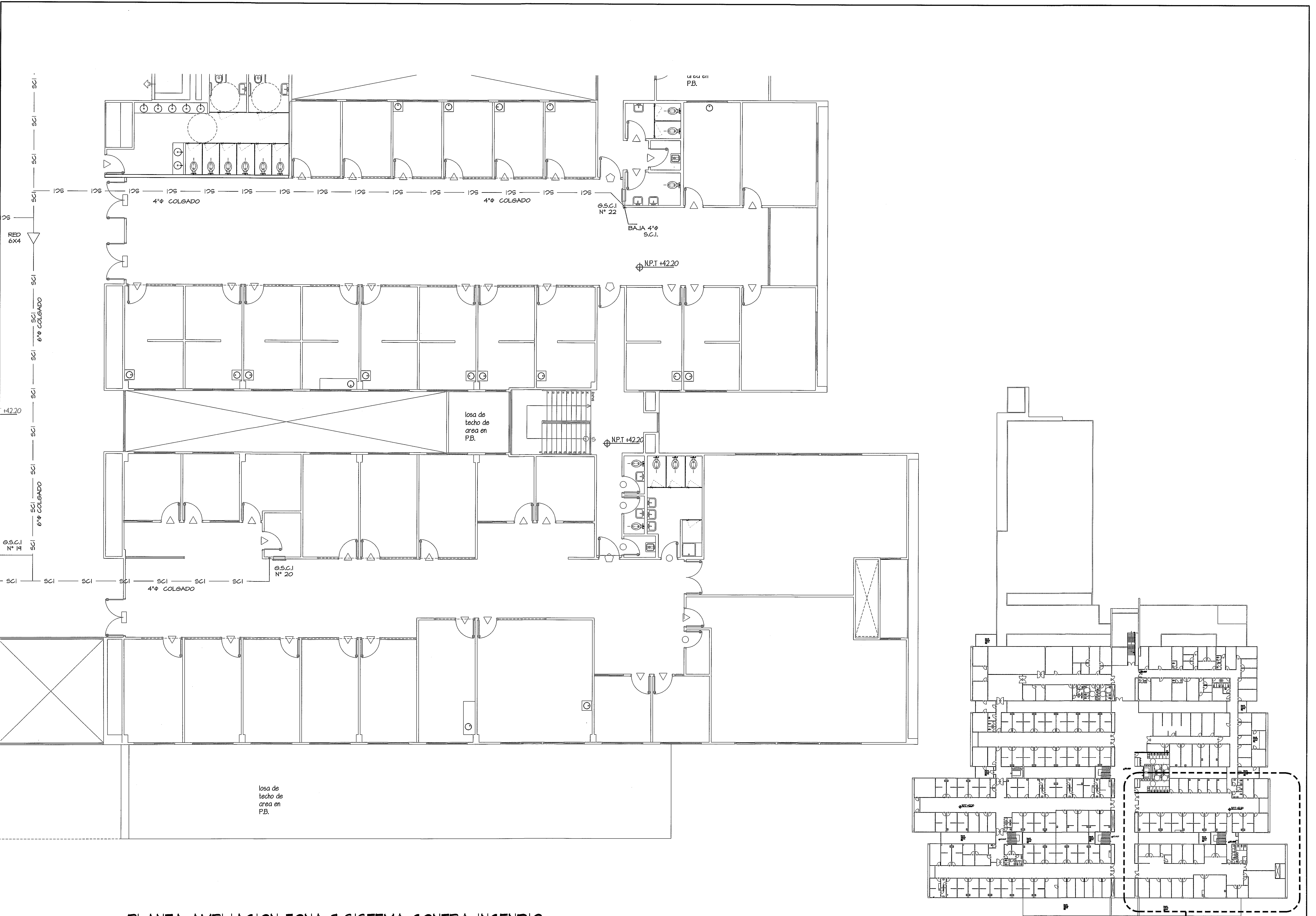
PLANTA AMPLIACION ZONA 9 SISTEMA CONTRA INCENDIO ESCALA 1:75
