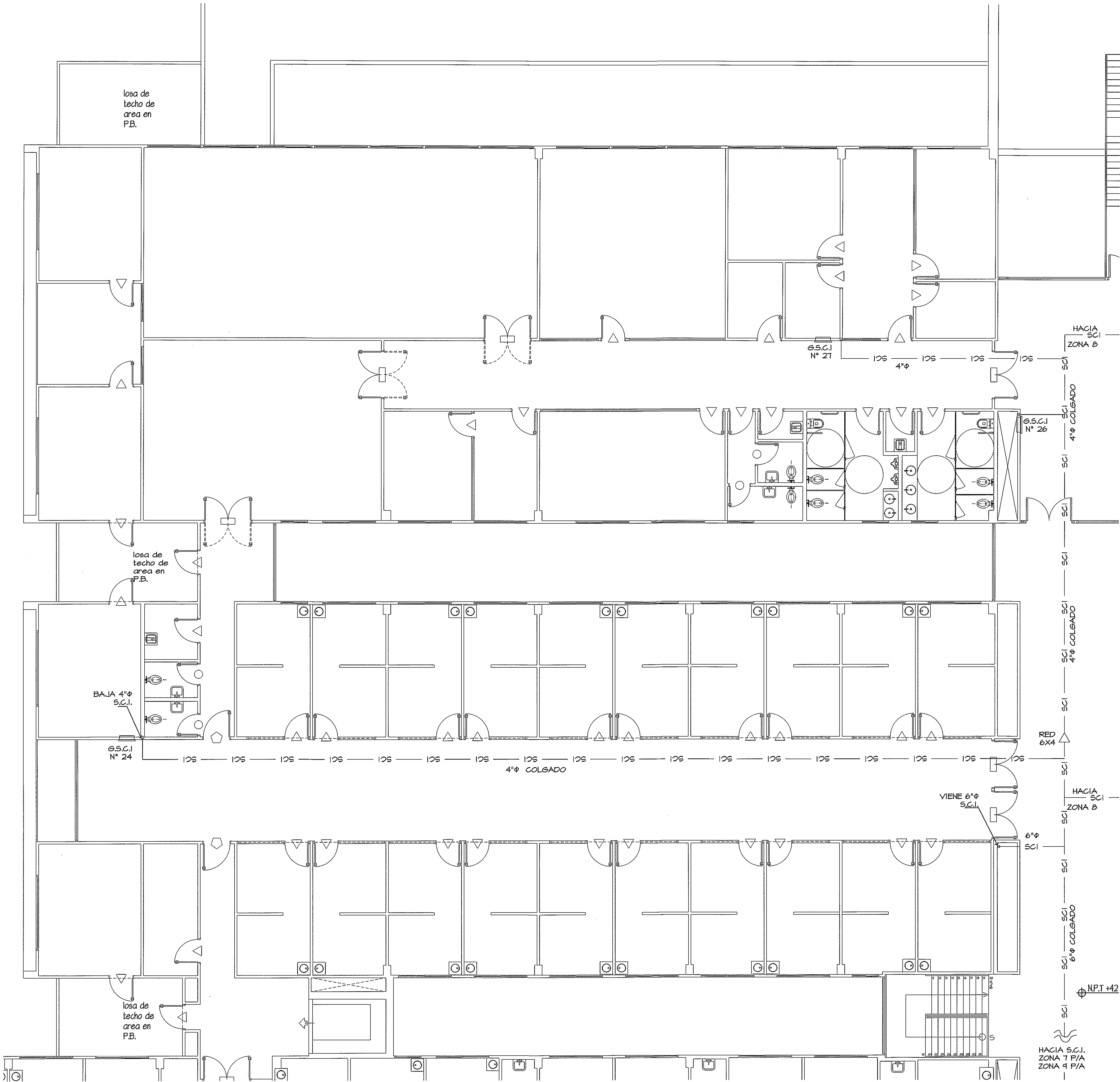
PLANTA AMPLIACION ZONA 6 SISTEMA CONTRA INCENDIO ESCALA 1:75
