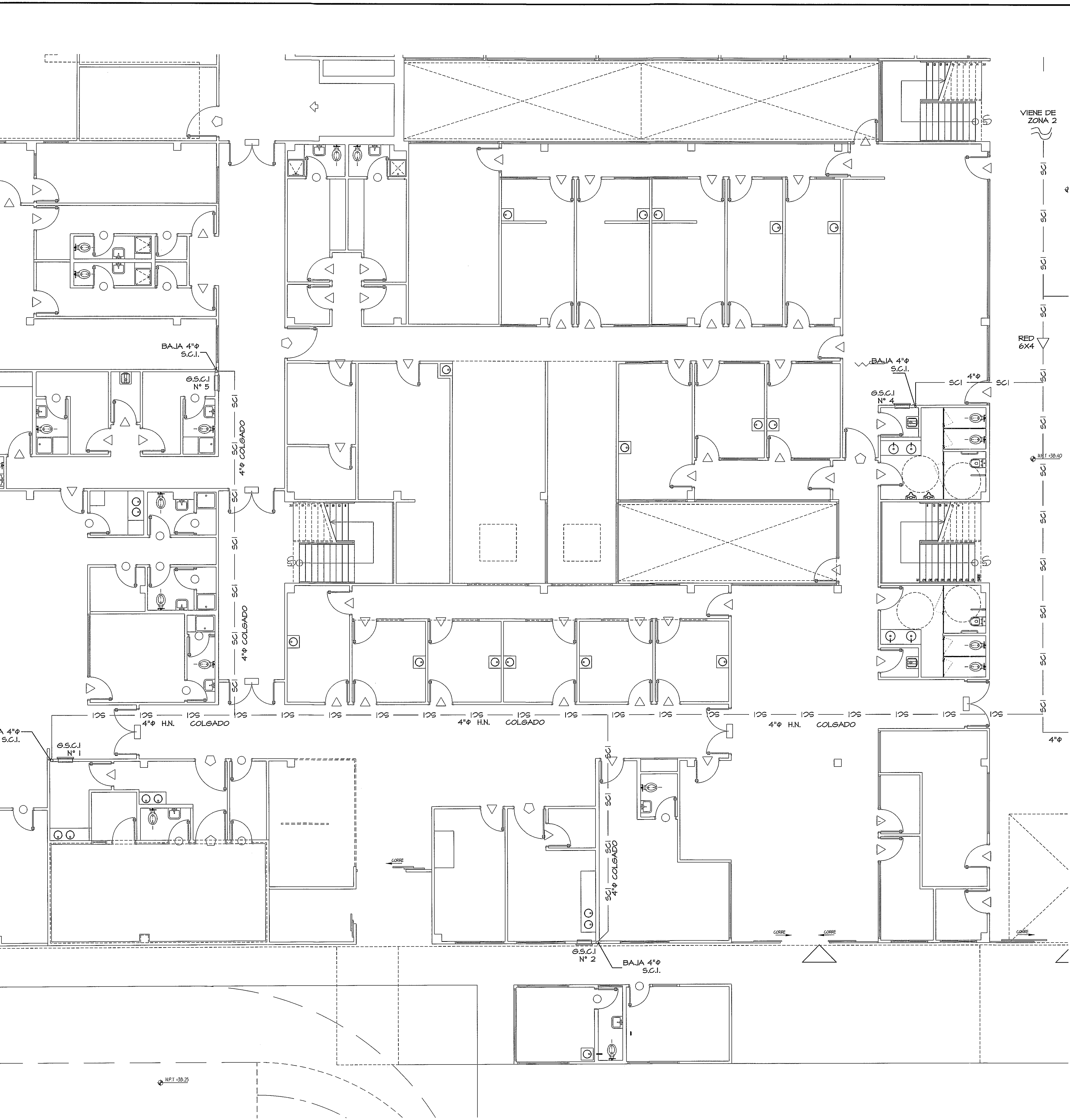
PLANTA AMPLIACION DE ZONA 3 SISTEMA CONTRA INCENDIO ESCALA 1:75
