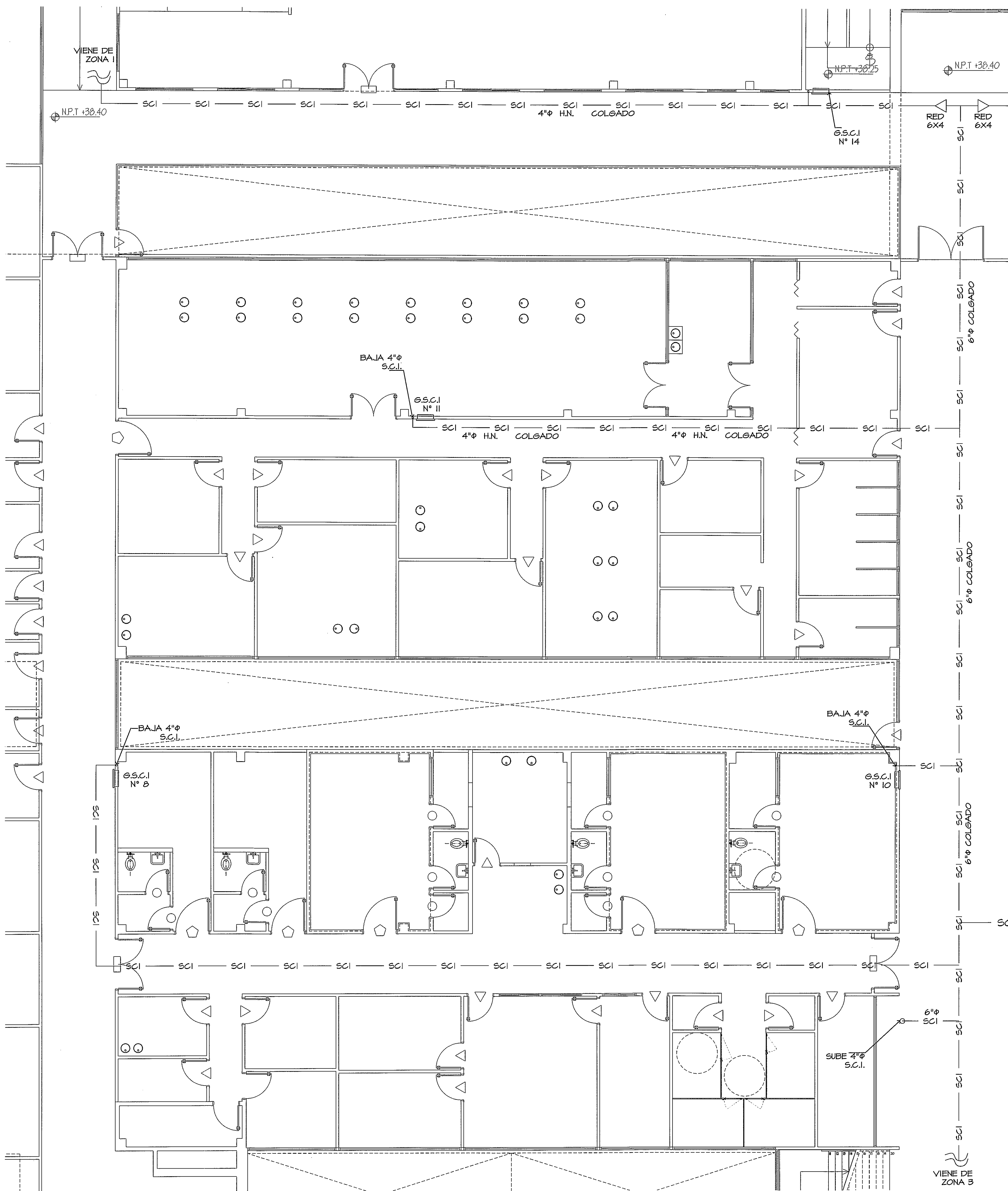
PLANTA AMPLIACION DE ZONA 2 SISTEMA CONTRA INCENDIO ESCALA 1:75
