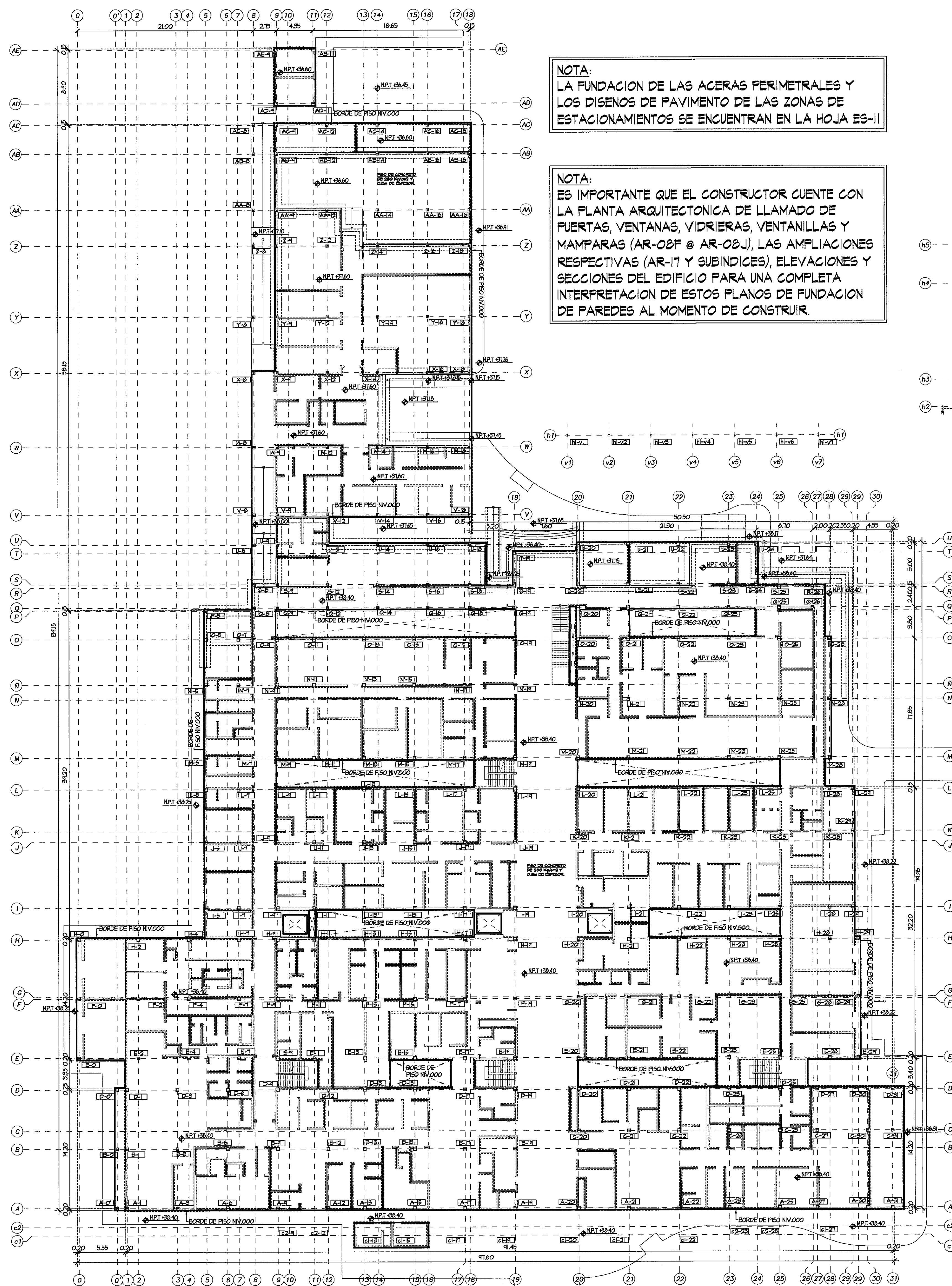
PLANTA DE CIMIENTOS DE PAREDES ESCALA 1:250
