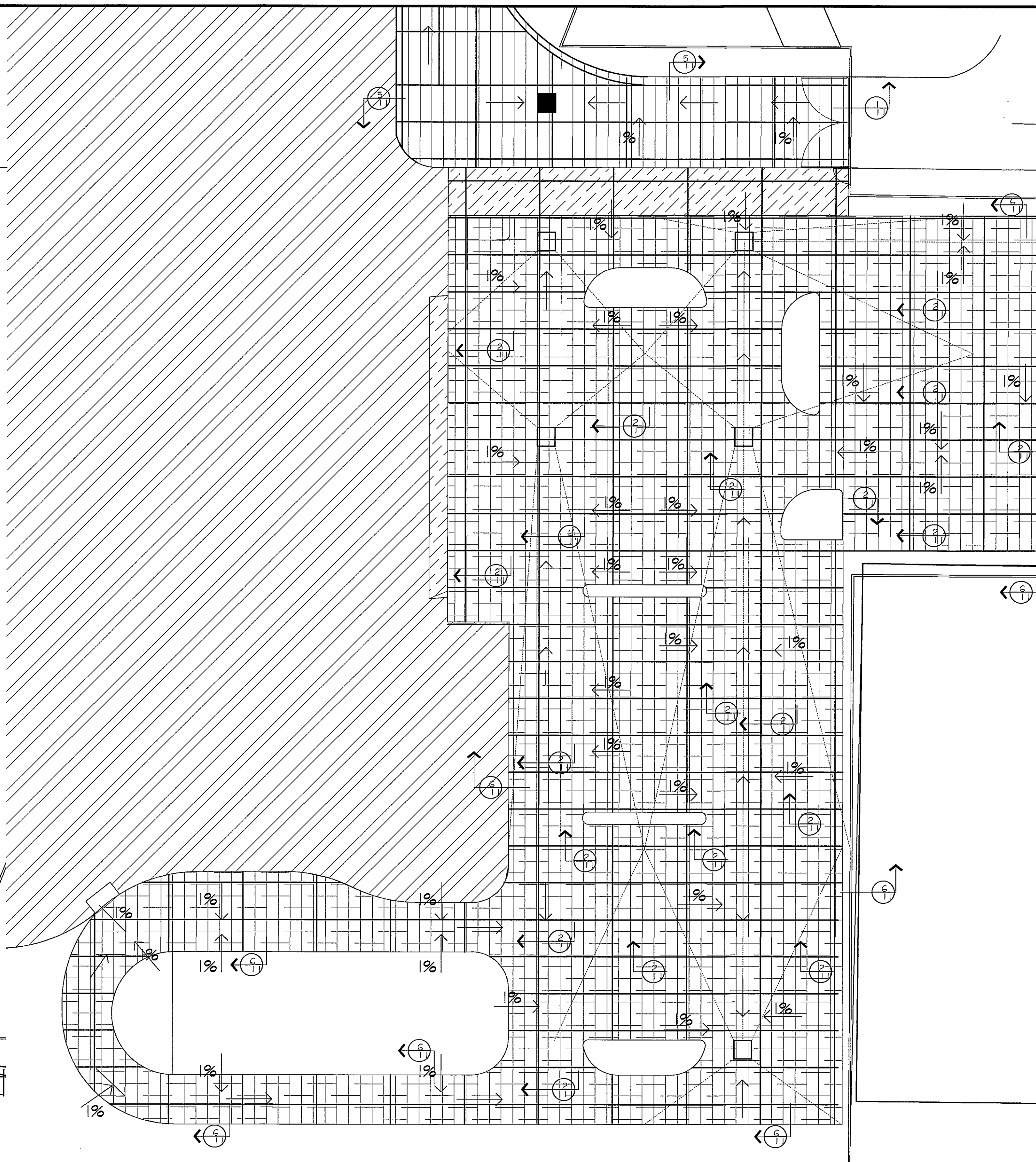
PLANTA - TIPOS DE PAVIMENTOS AREA 2 ESCALA 1:200
