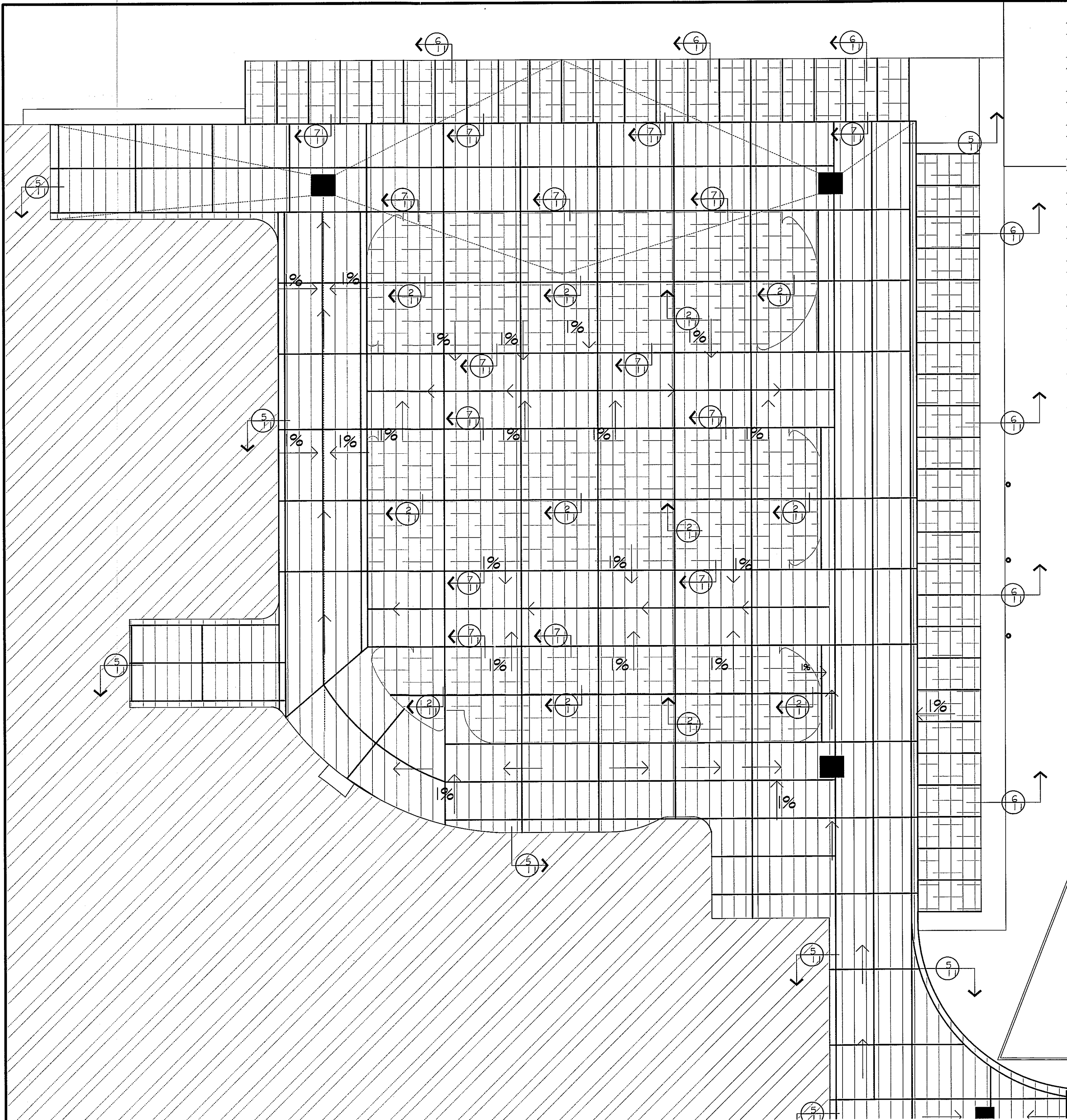
PLANTA - TIPOS DE PAVIMENTOS AREA 1 ESCALA 1:200
