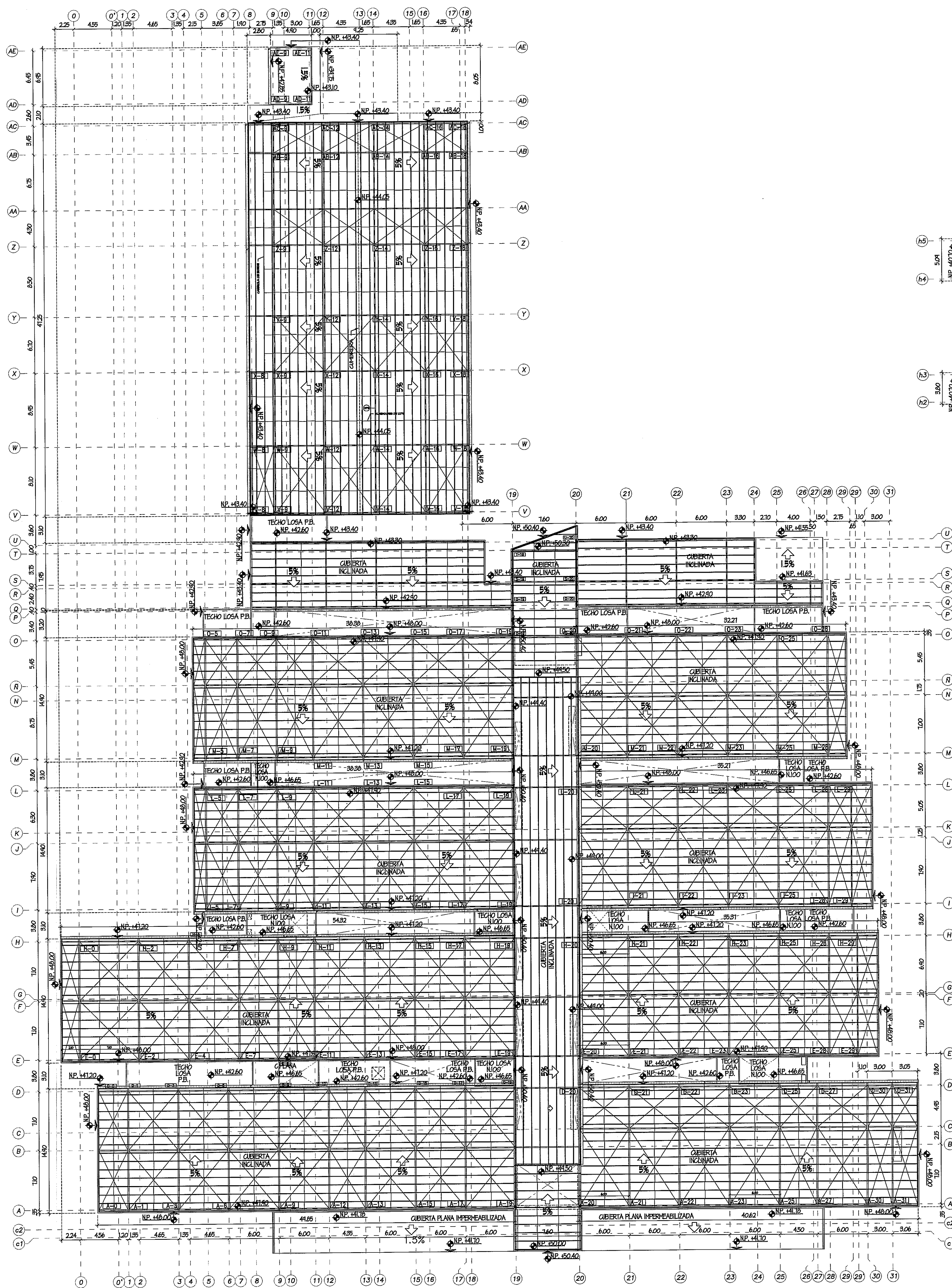
PLANTA GENERAL DE TECHOS ESCALA 1:250
