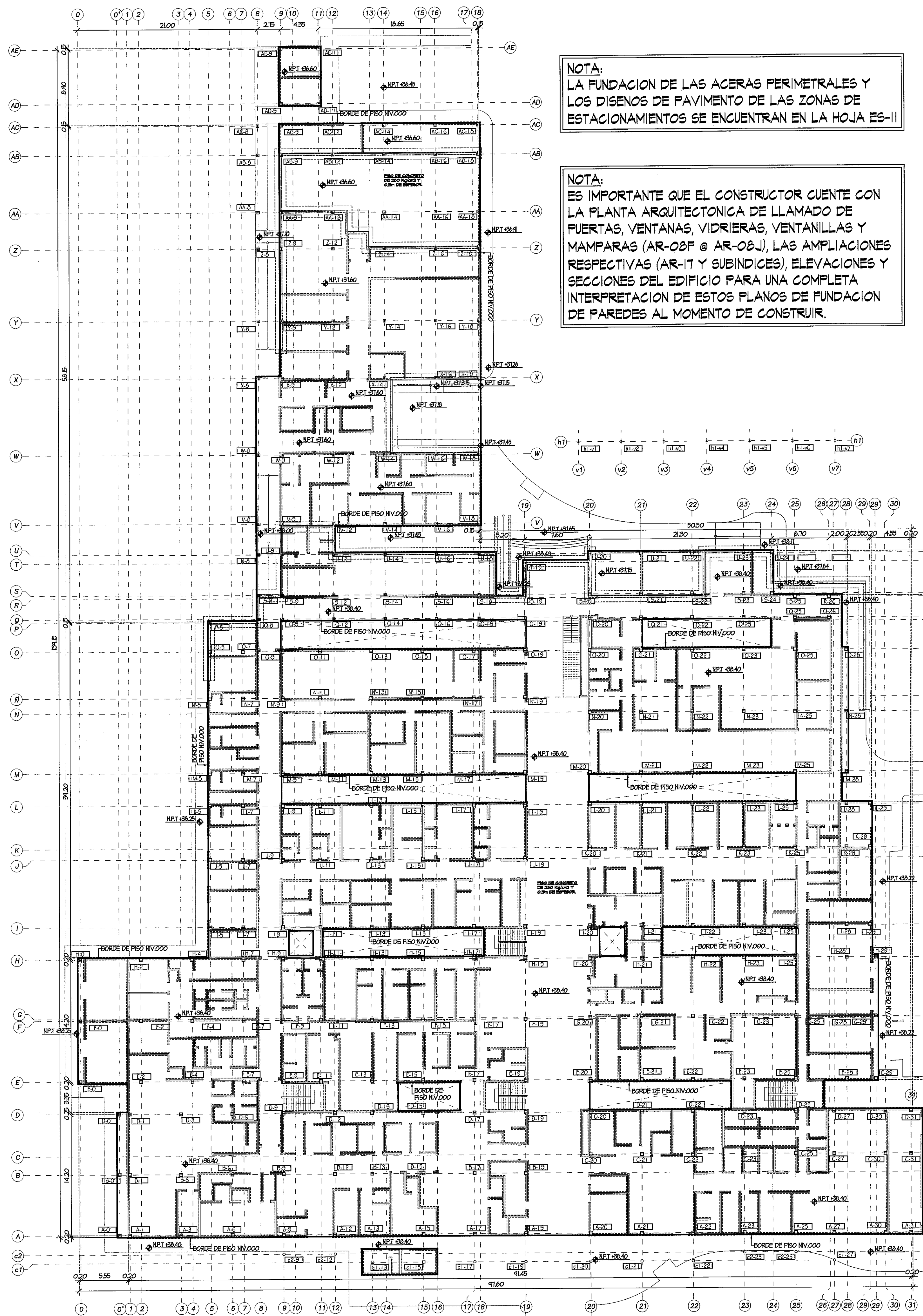
PLANTA DE CIMIENTOS DE PAREDES ESCALA 1:250
