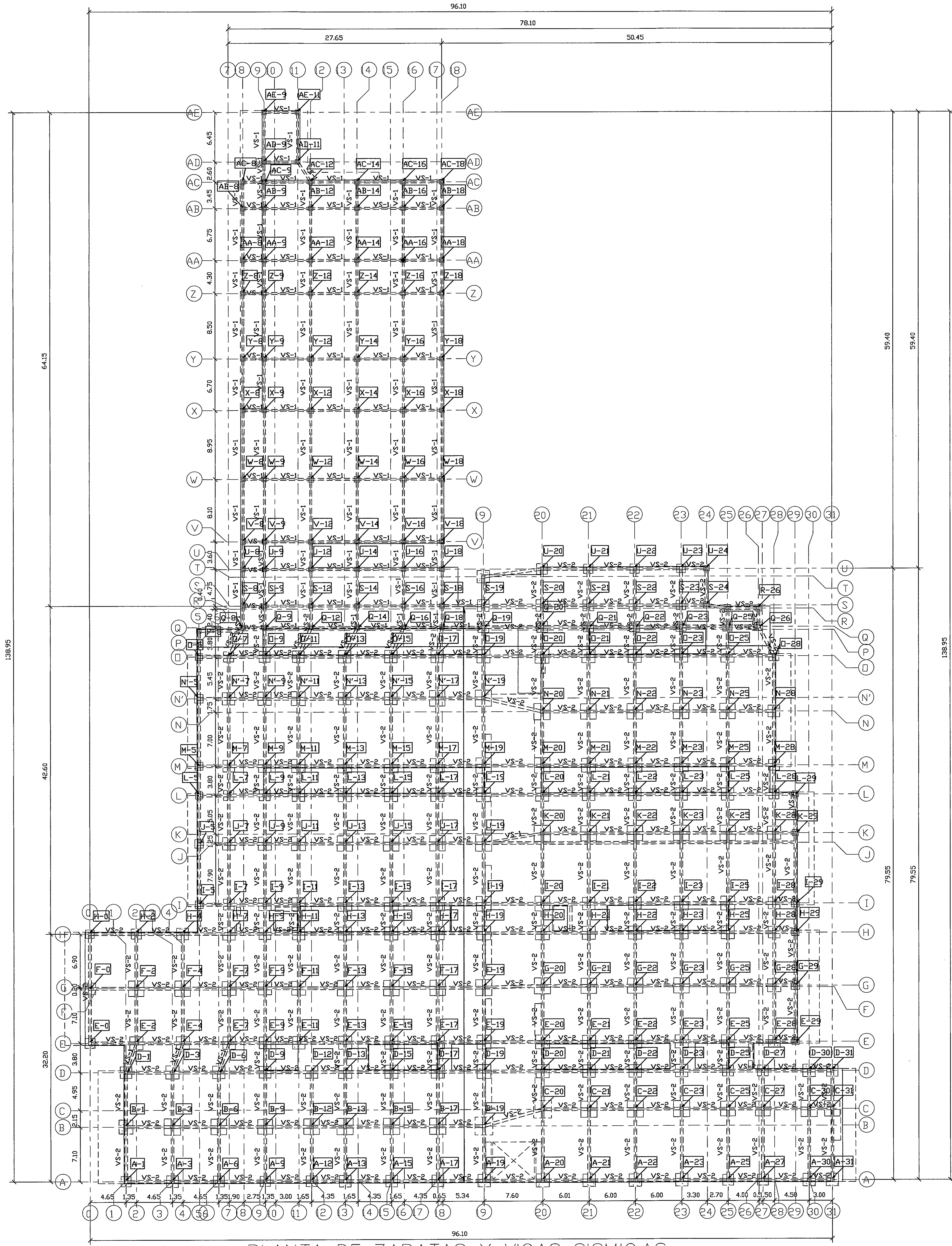
1 PLANTA DE ZAPATAS Y VIGAS SISMICAS ES-2 1 : 250
