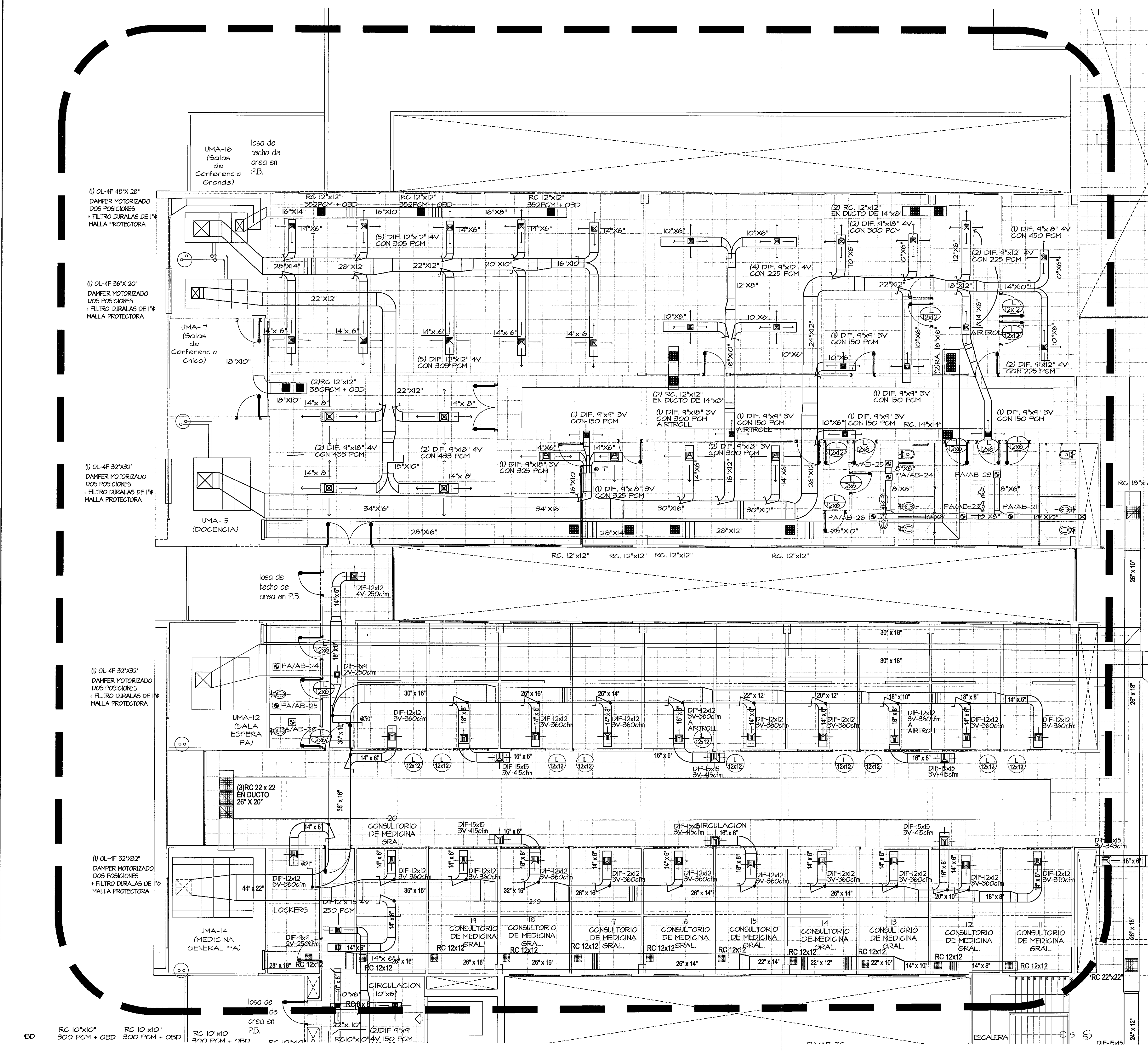
PLANTA DE AIRE ACONDICIONADO-ZONA #6 PLANTA ALTA ESCALA.- 1/75
