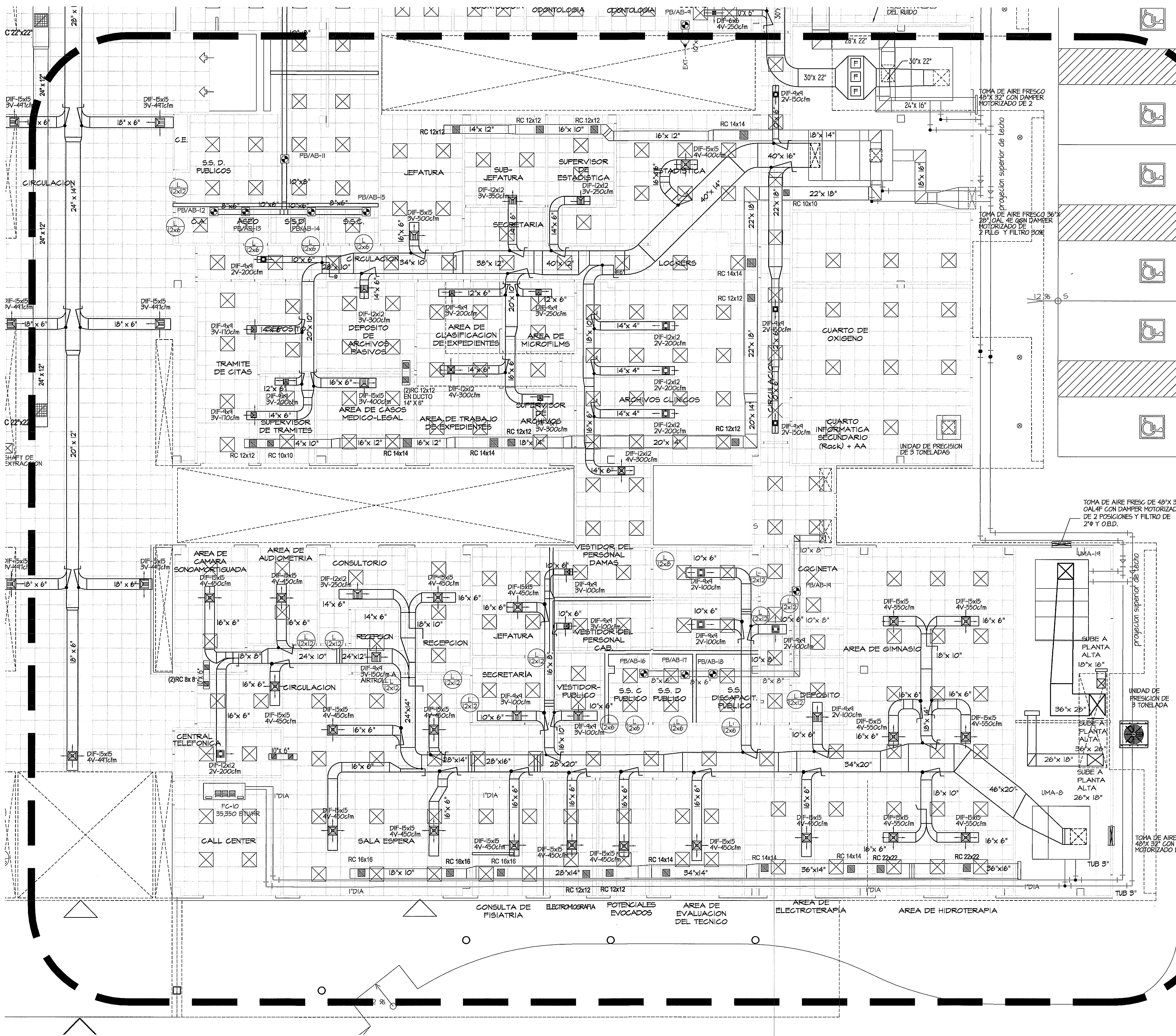
PLANTA DE AIRE ACONDICIONADO-ZONA #2 PLANTA BAJA
