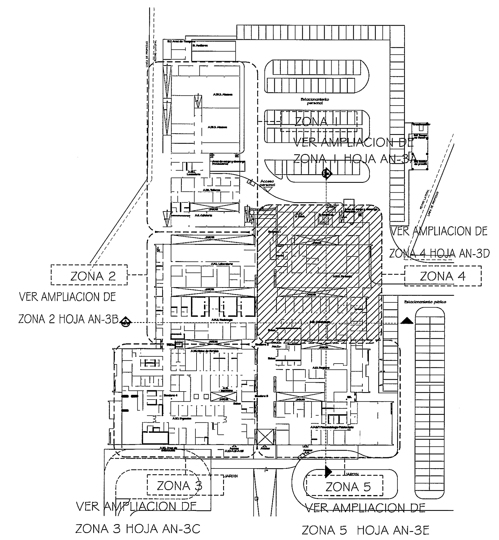
GUIA DE AMPLIACIONES POR ZONAS ESCALA.- 1/750 PLANTA BAJA (NIVEL 000, -050, -100)
