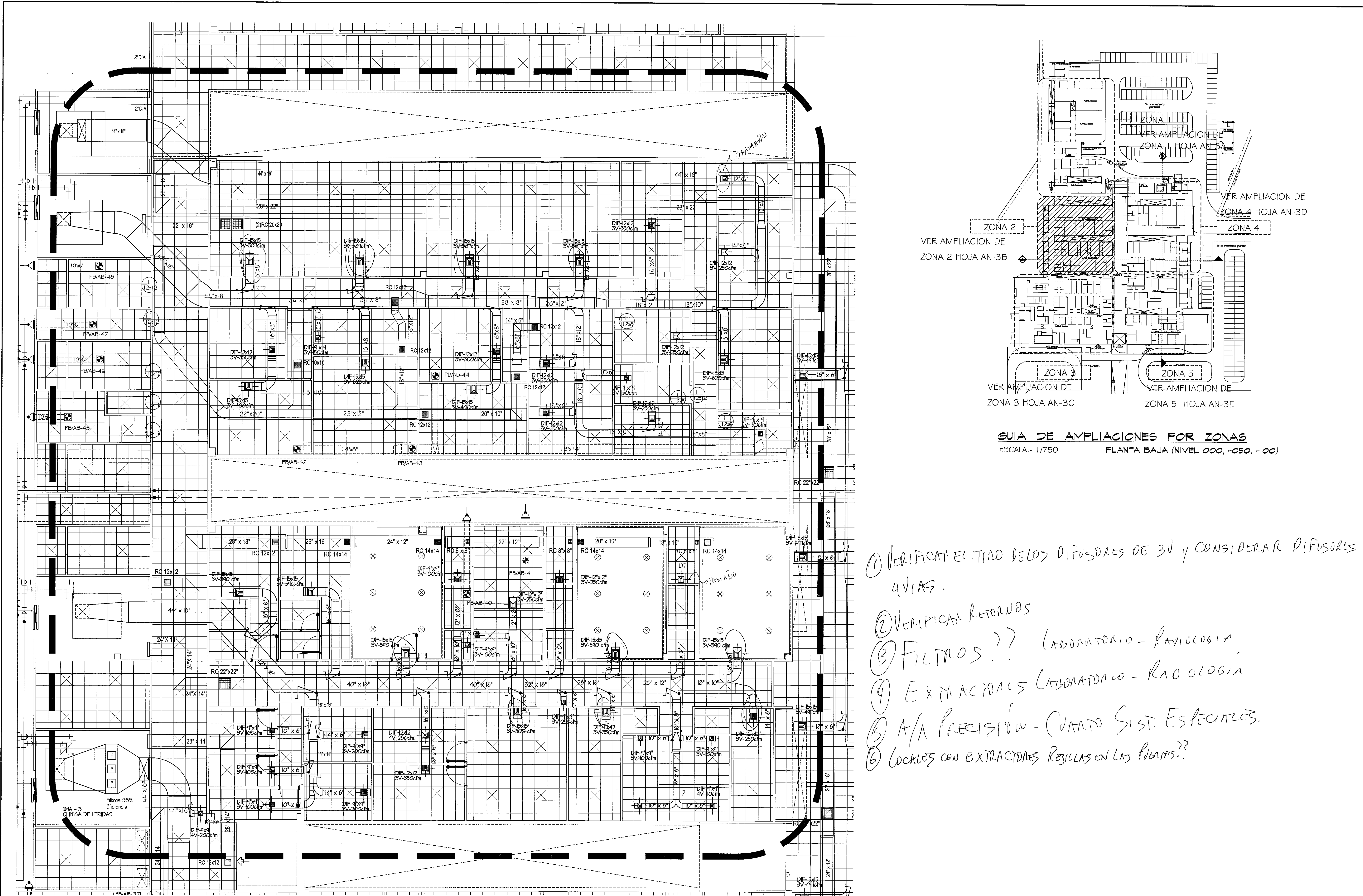
PLANTA DE AIRE ACONDICIONADO-ZONA #2 PLANTA BAJA ESCALA.- 1/75
