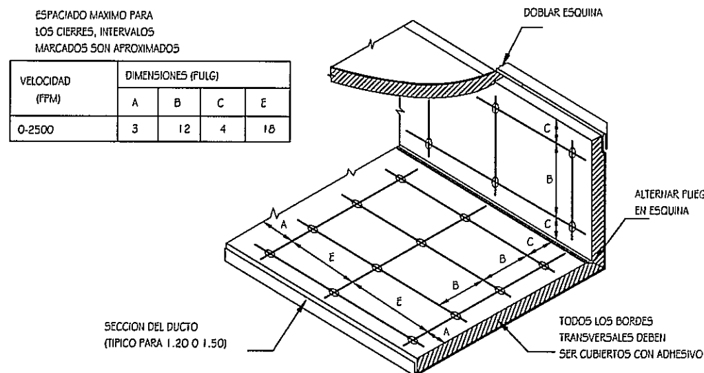
DETALLE DE INSTALACION DEL AISLAMIENTO ACUSTICO SIN ESCALA
