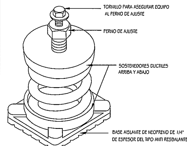
AISLADOR DE UNIDADES MANEJADORAS - TIPO SLF SIN ESCALA
