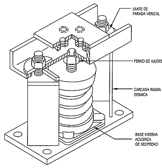
AISLADOR DE ENFRIADORES DE LIQUIDO - TIPO SLR SIN ESCALA
