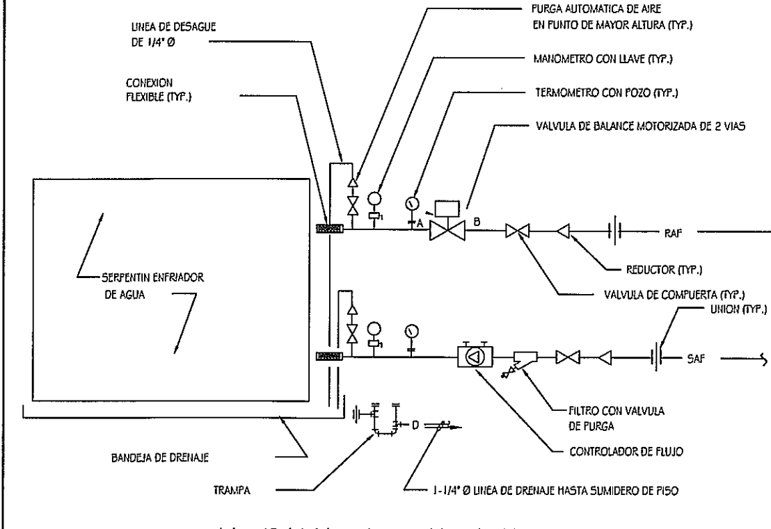
DIAGRAMA DE CONEXION DE LAS MANEJADORAS DE AIRE (UMA) SIN ESCALA
