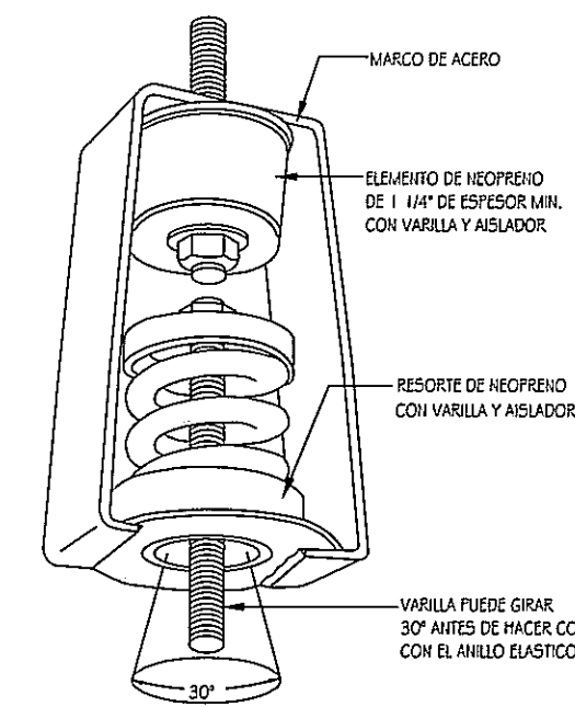
SOPORTE DE TUBERIA DE AGUA COND. - TIPO SON CON RESORTE Y COLADOR DE REPOLENDO
