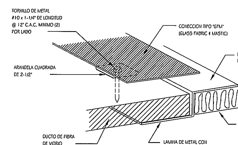
DETALLE DE CAMBIO DE DUCTO DE FIBRA DE VIDRIO A DUCTO DE METAL SIN ESCALA
