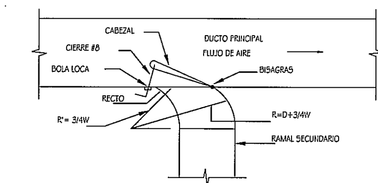
DETALLE DE CONEXION SECUNDARIA DE DUCTOS SIN ESCALA
