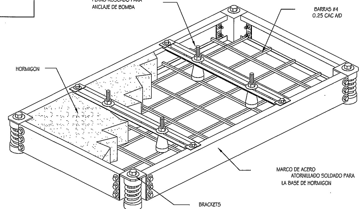
BASE ACERO PARA BOMBAS - TIPO BMK SIN ESCALA
