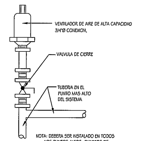
DETALLE DE VENTILADOR AUTOMATICO SIN ESCALA
