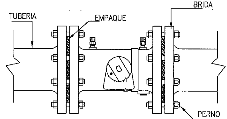
DETALLE DE VALVULA DE BALANCE EN TUBERIA SIN ESCALA
