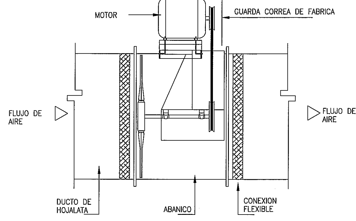
DETALLE INSTALACION DE ABANICO SIN ESCALA
