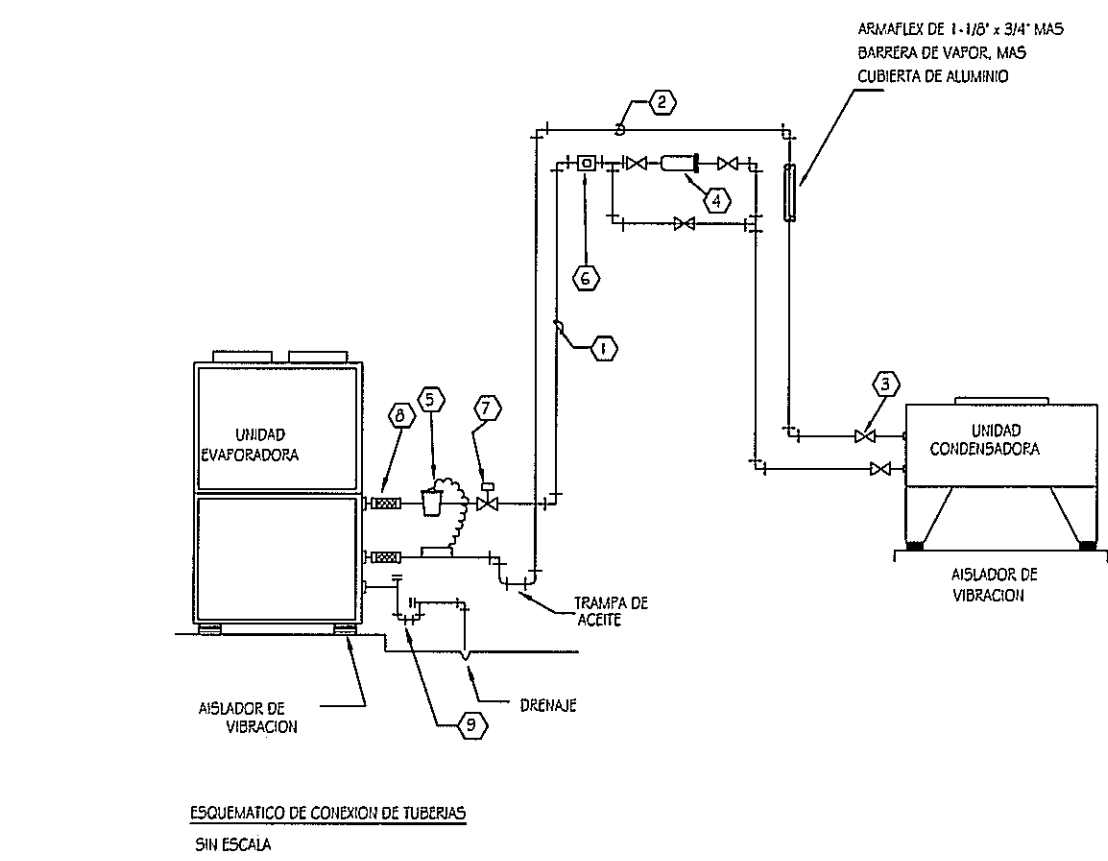
ESQUEMA DE CONEXION DE TUBERIA SIN ESCALA
