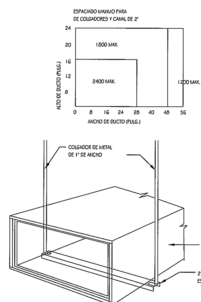
DETALLE DE COLGADOR DE DUCTO SIN ESCALA
