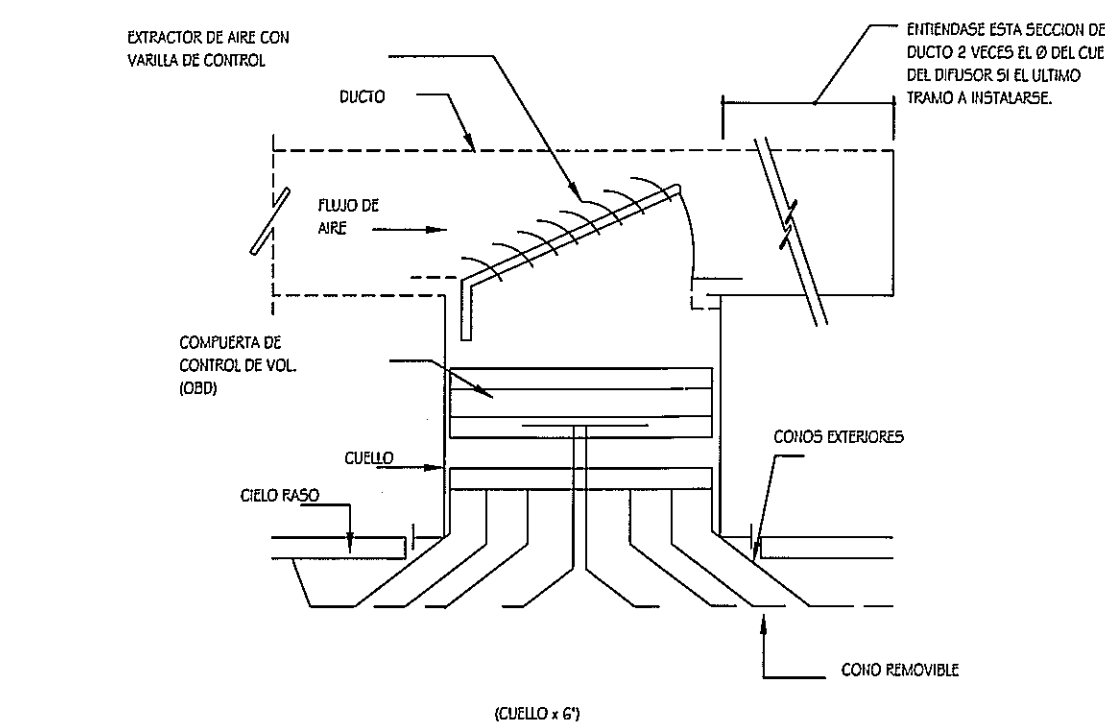
DET. DE INSTALACION DE DIFUSOR SIN ESCALA
