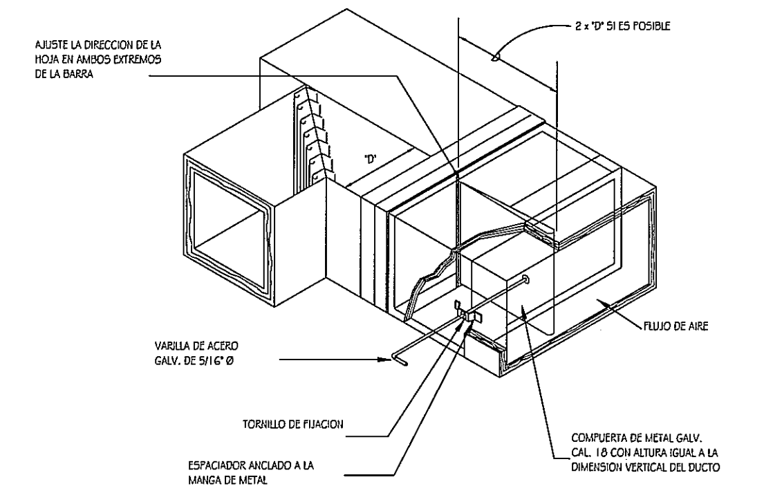
DETALLE DE COMPUERTA CON SEPARADOR HORIZONTAL DE AIRE (TIPICO) SIN ESCALA
