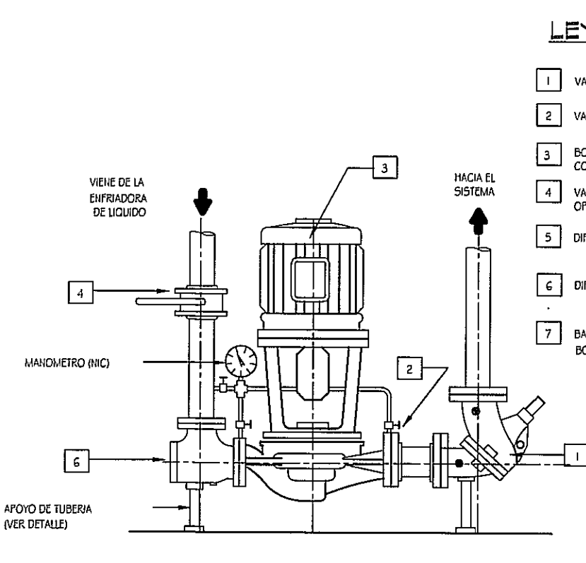
DETALLE DE CONEXION DE BOMBA (TIPICO) SIN ESCALA
