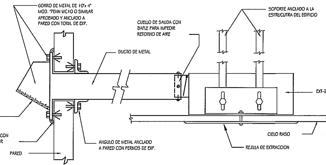
DETALLE DE INSTALACION DE EXTRACTOR DE AIRE SIN ESCALA
