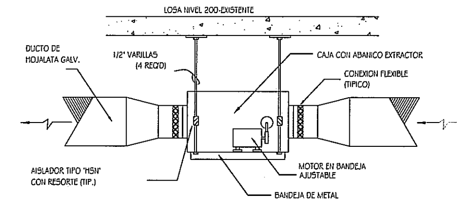
DETALLE DE INSTALACION DE ASPIRADOR EXTRACTOR SIN ESCALA
