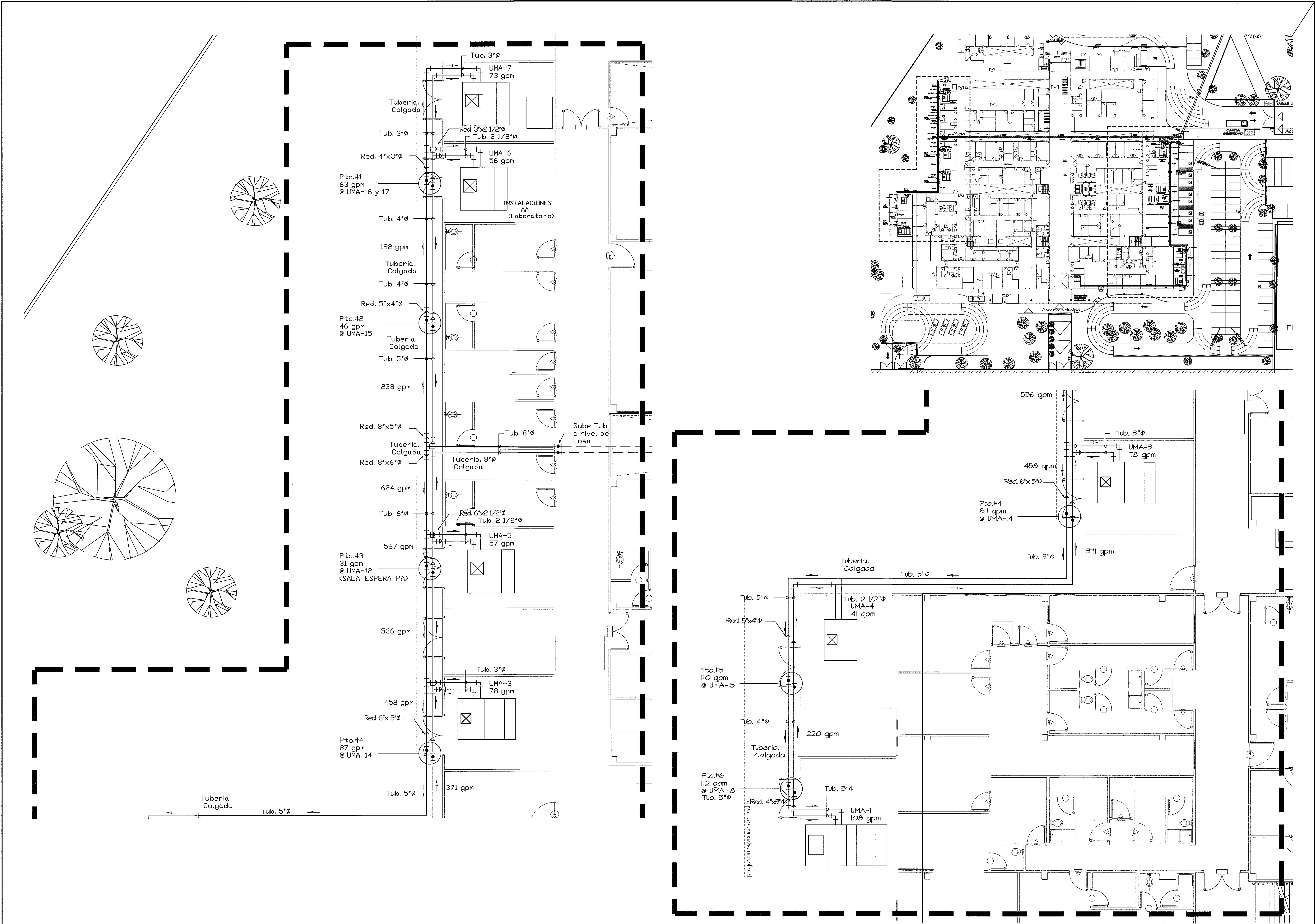
PLANTA BAJA TUBERIAS DE AGUA FRIA ZONA-I ESCALA:- 1/75
