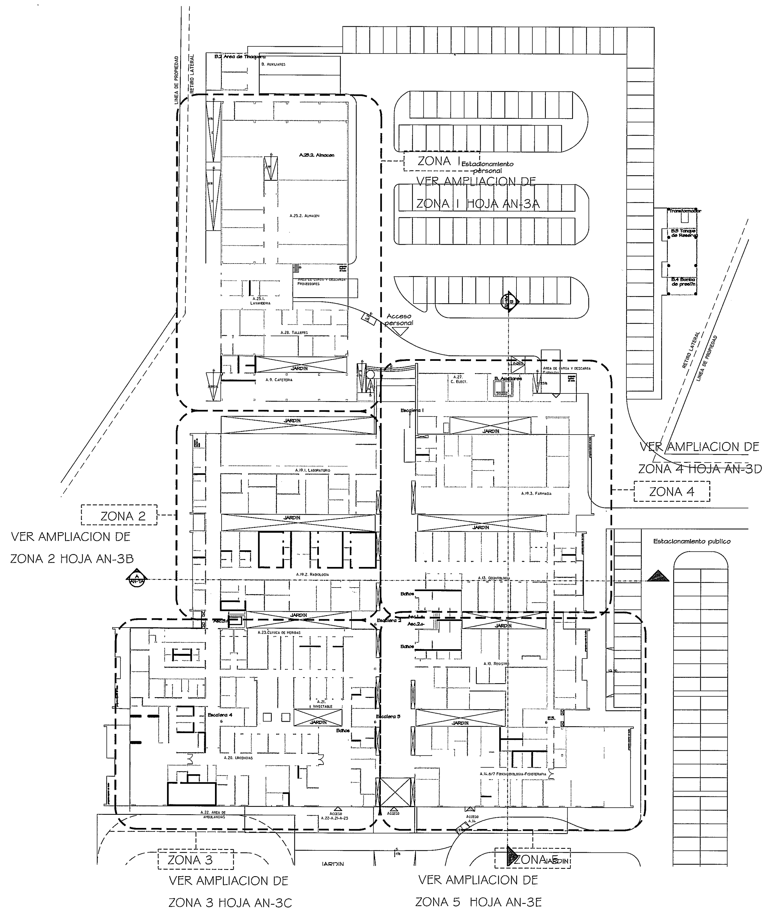
GUIA DE AMPLIACIONES POR ZONAS ESCALA.- 1/400 PLANTA BAJA (NIVEL 000, -050, -100)
