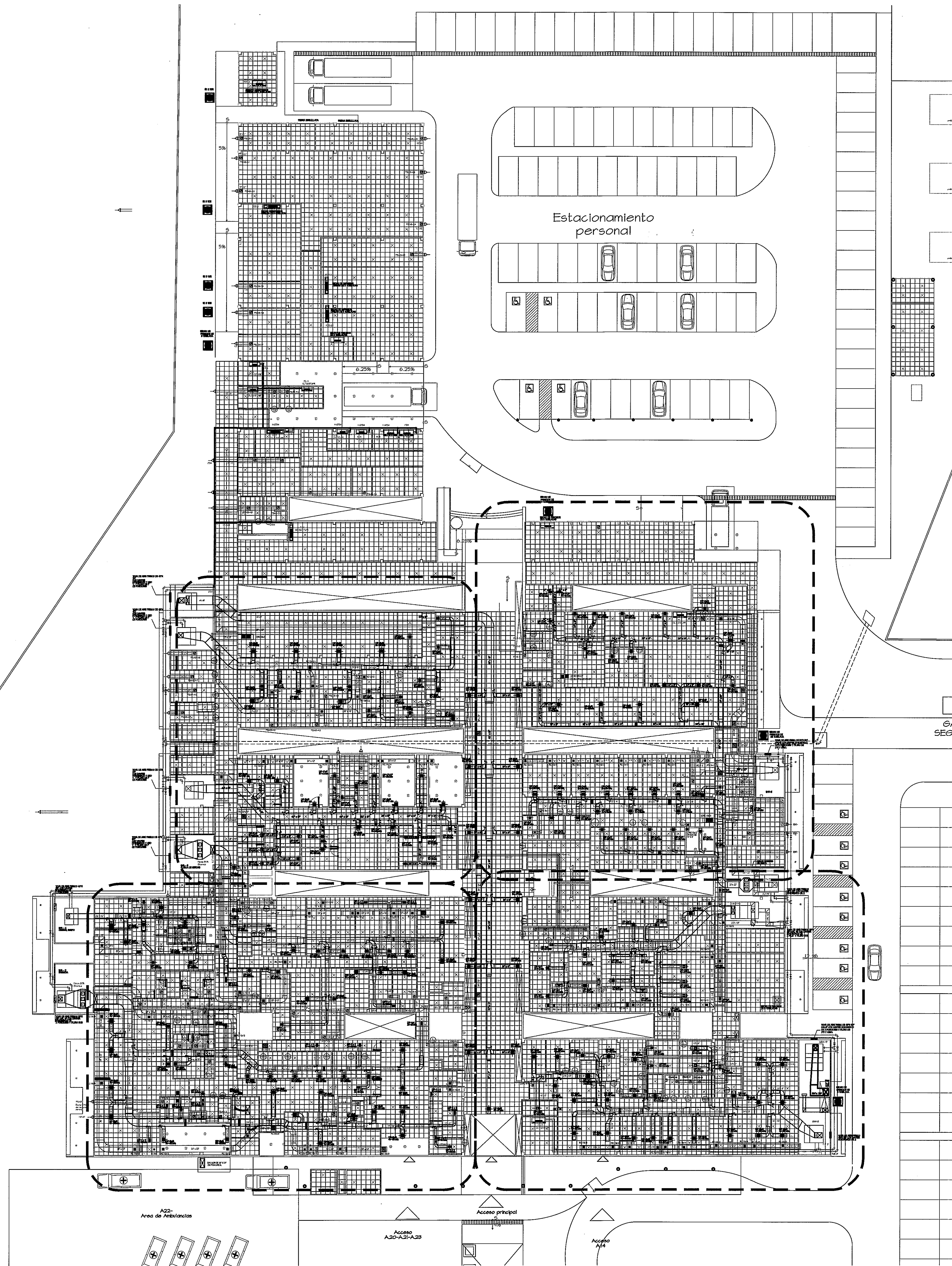
PLANTA BAJA ARQUITECTONICA NIVEL 000, -050 Y -100) ESCALA.- 1/250
