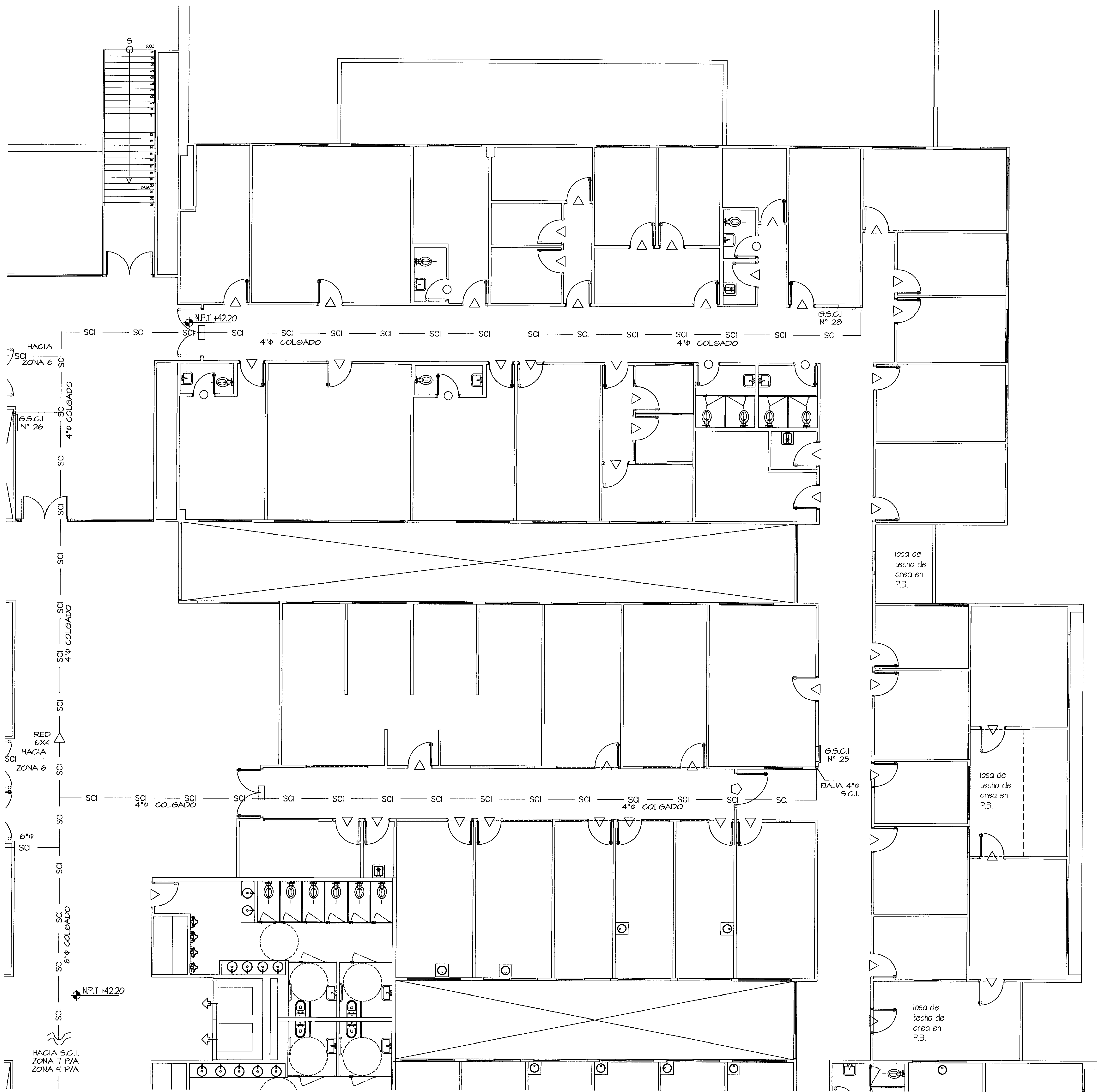
PLANTA AMPLIACION ZONA 8 SISTEMA CONTRA INCENDIO ESCALA 1:75
