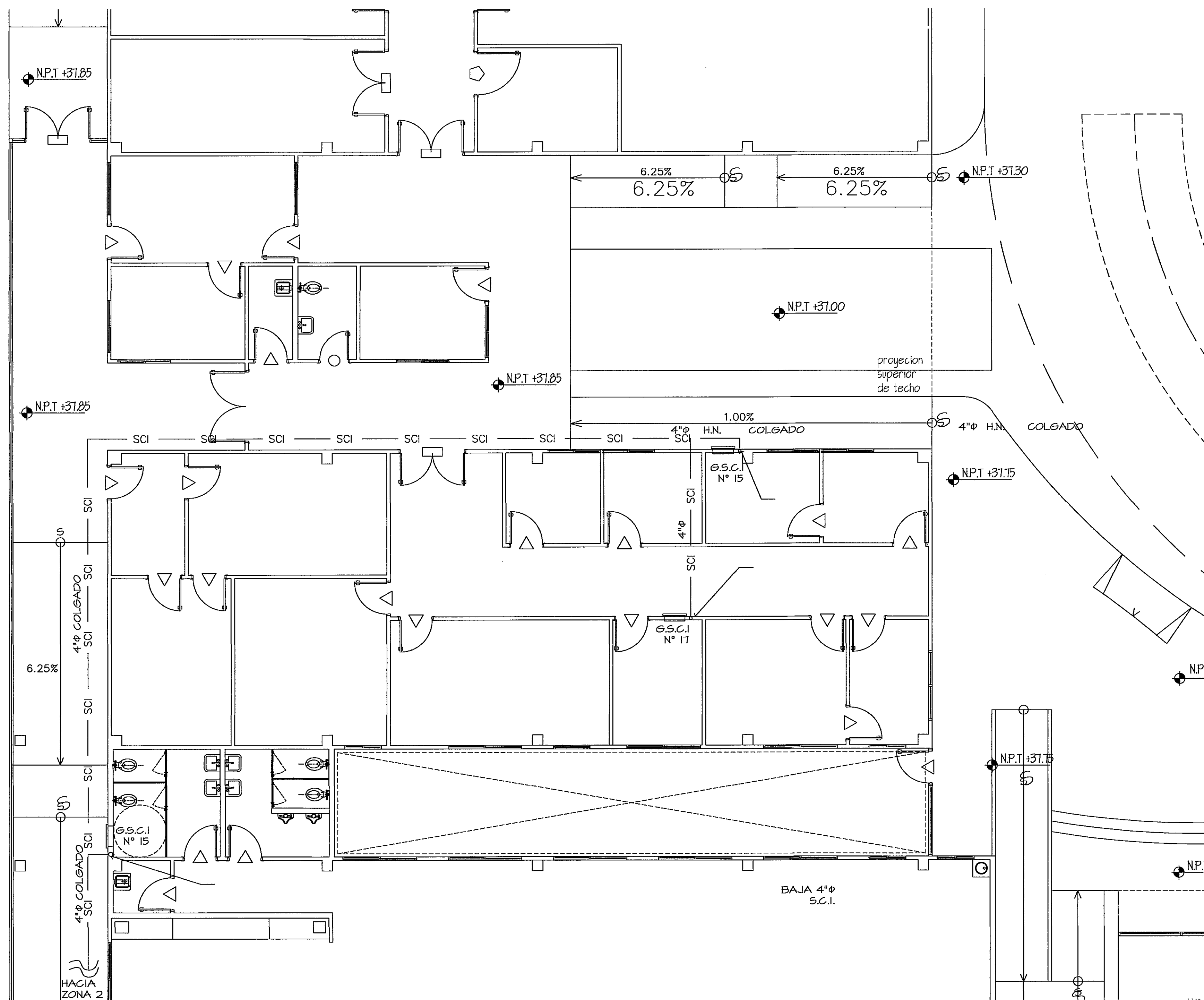
PLANTA AMPLIACION DE ZONA I SISTEMA CONTRA INCENDIO ESCALA 1:75
