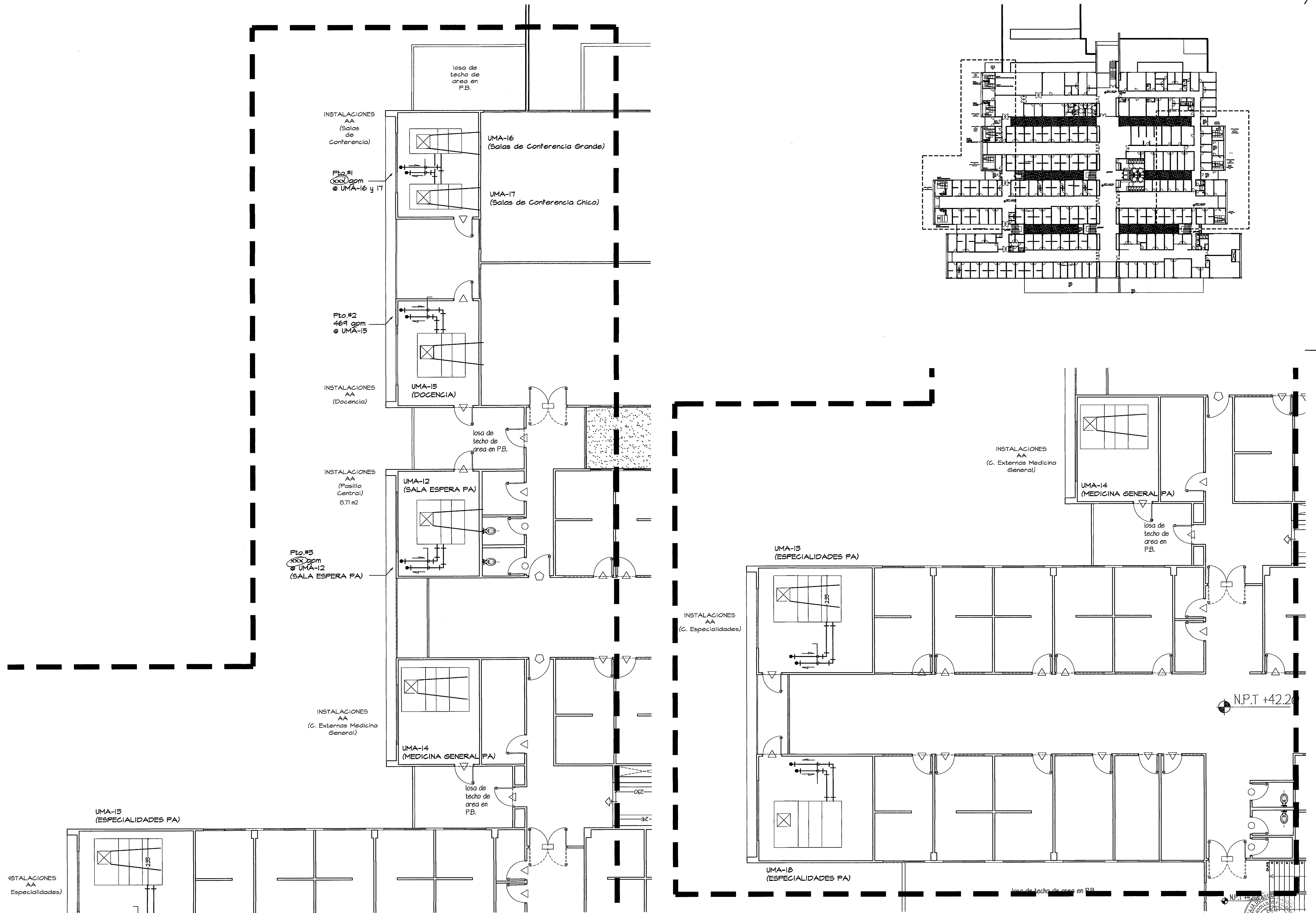
PLANTA BAJA TUBERIAS DE AGUA FRIA ZONA-2 ESCALA.- 1/75
