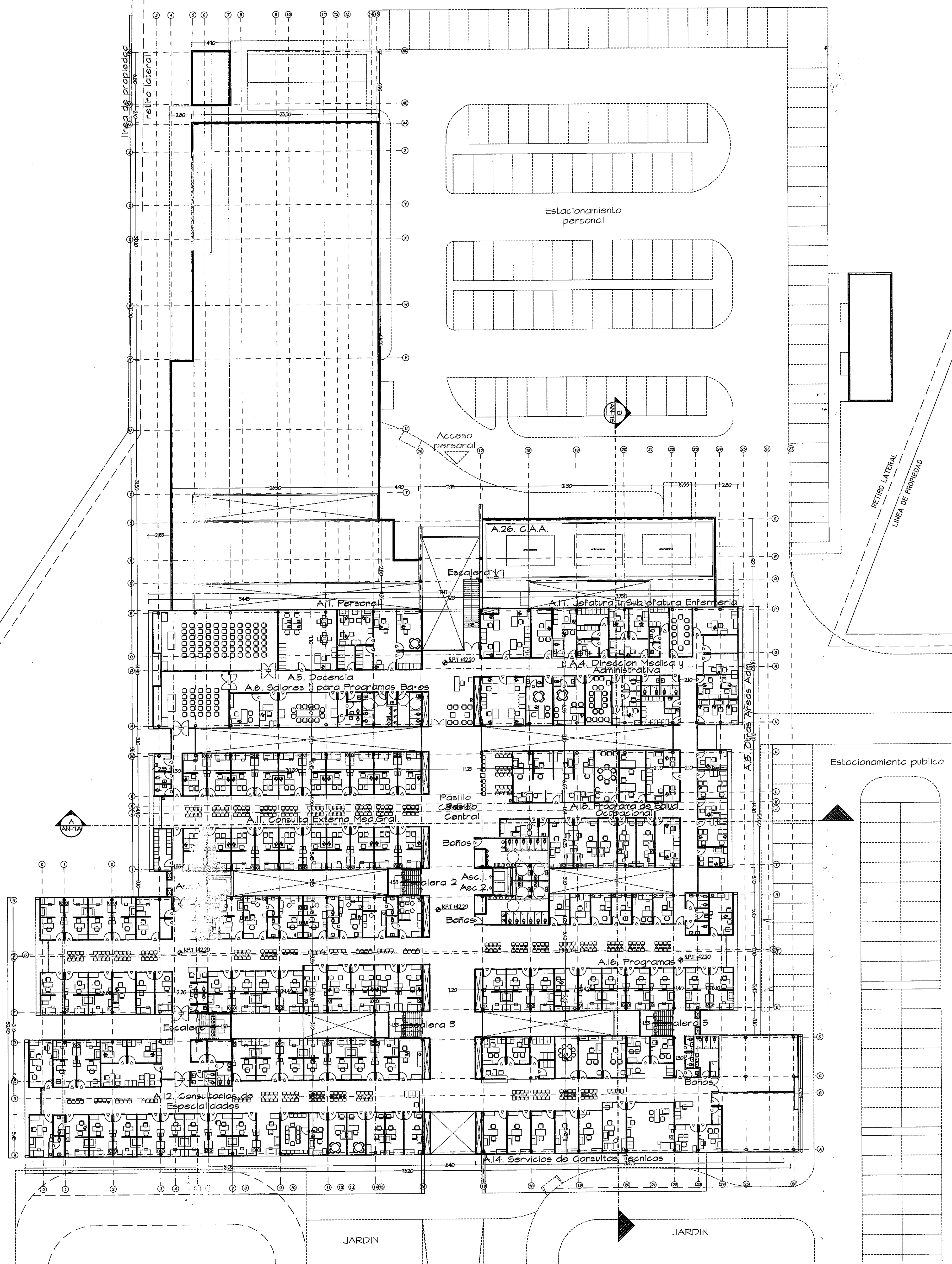
PLANTA ALTA ARQUITECTONICA NIVEL 100) ESCALA.- 1/250
