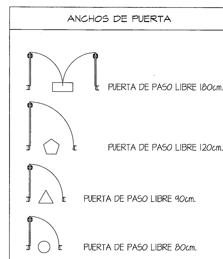
AMPLIACION DE ZONA 2 PLANTA BAJA ESCALA.- 1/75
