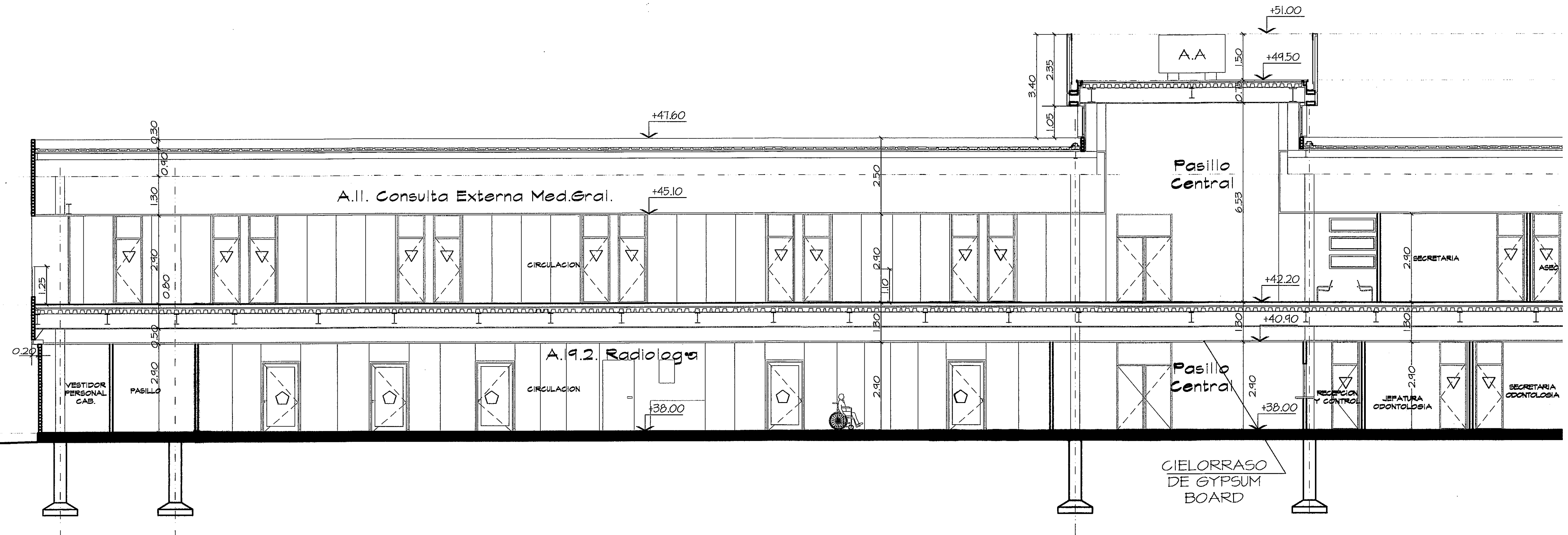
SECCION TRANSVERSAL ampliacion lado A esc 1:75
