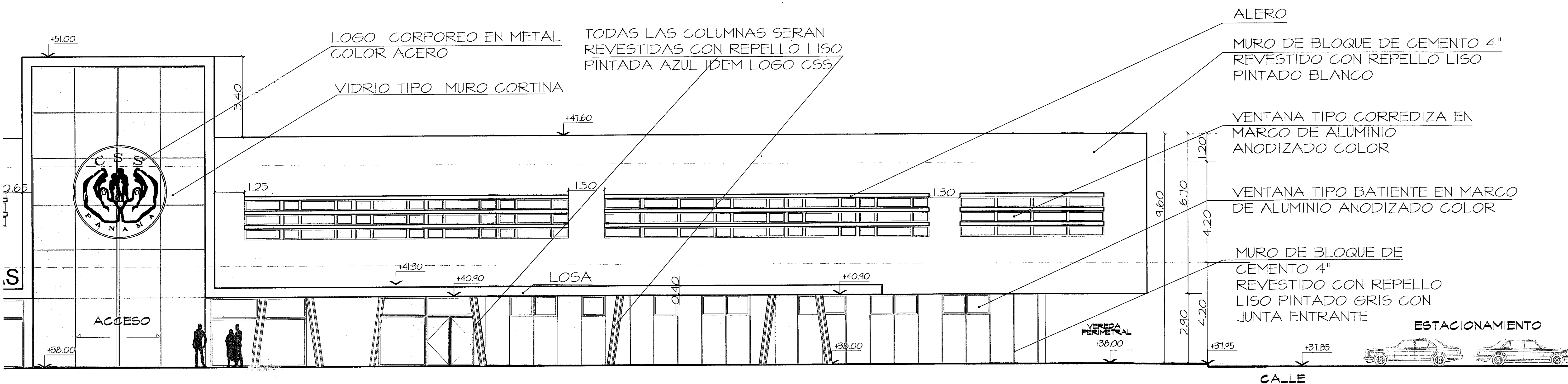
CONTINUA ELEVACION FRONTAL LADO "A" EN HOJA AN-6A
