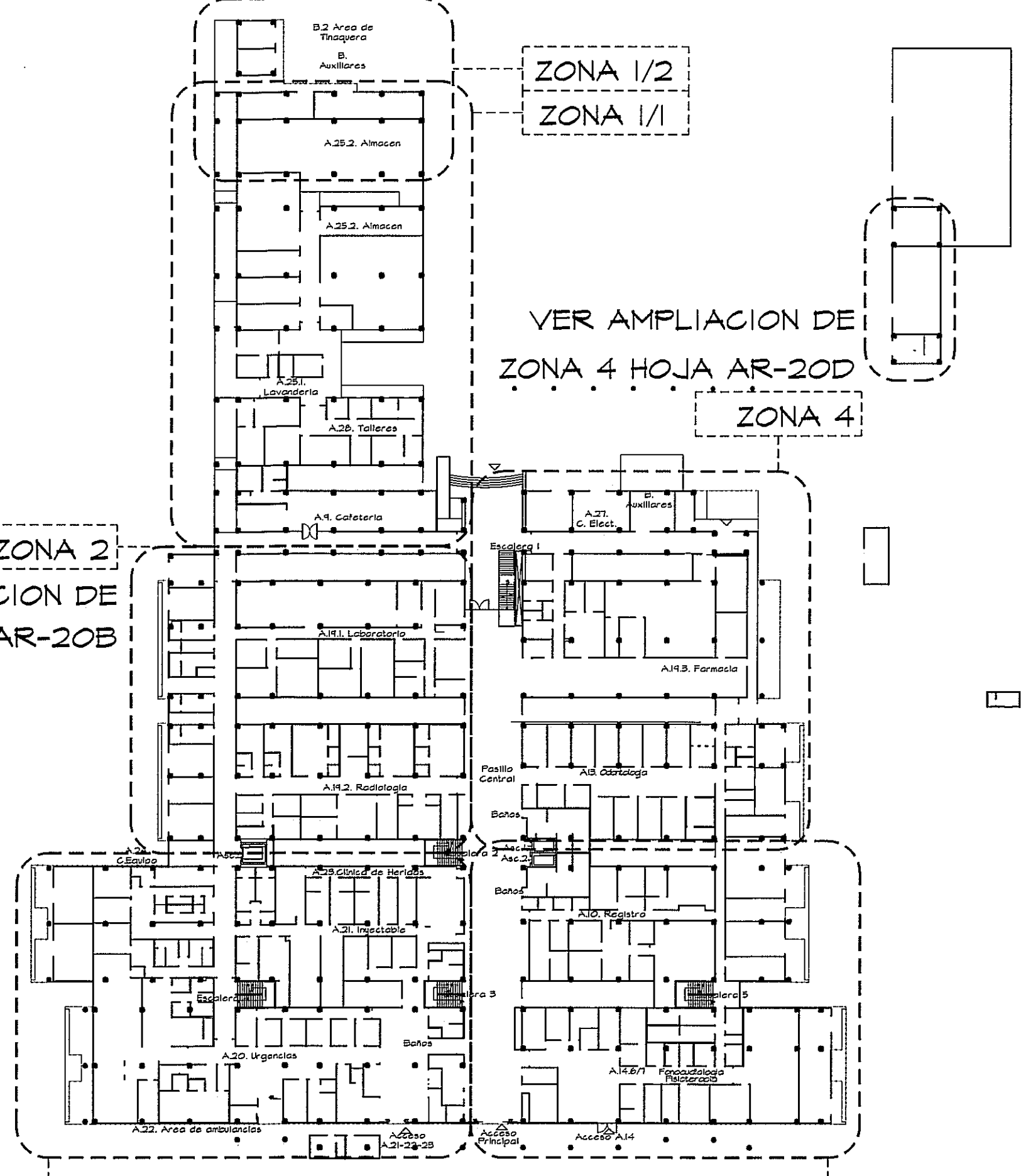
GUIA DE AMPLIACIONES POR ZONAS ESCALA.- 1/800 PLANTA BAJA
