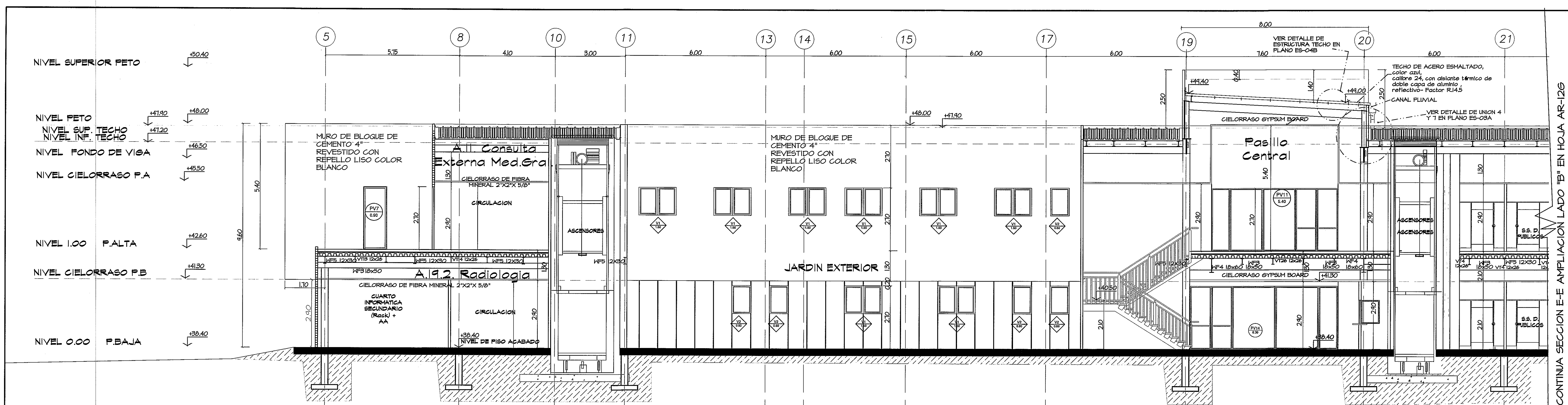
SECCION E-E ampliacion lado A ESC. 1:75
