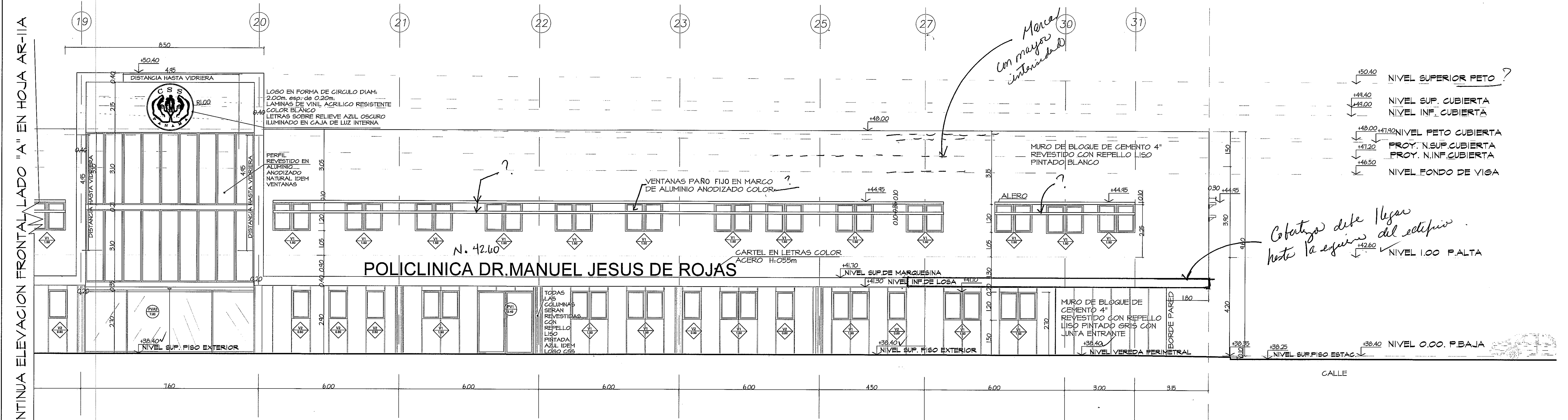
ELEVACION FRONTAL-AMPLIACION LADO "B" ESC. 1:75
