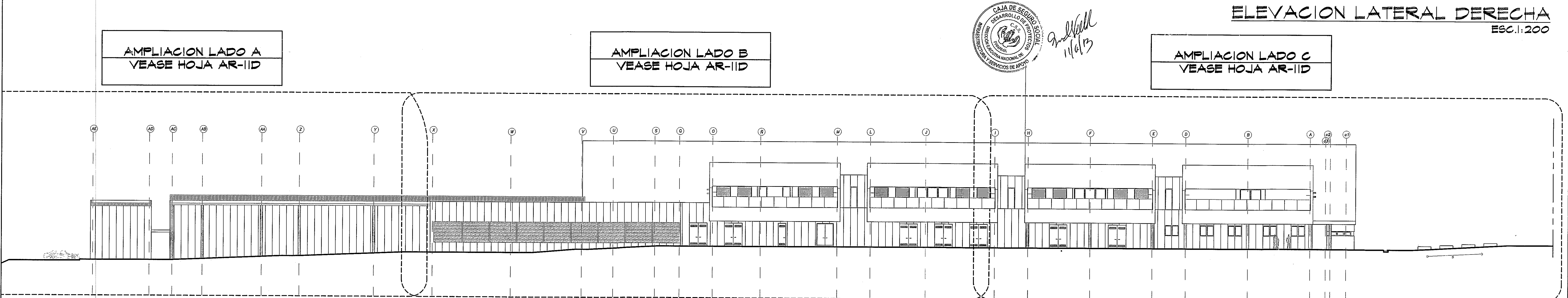
ELEVACION LATERAL IZQUIERDA ESC. 1:200
