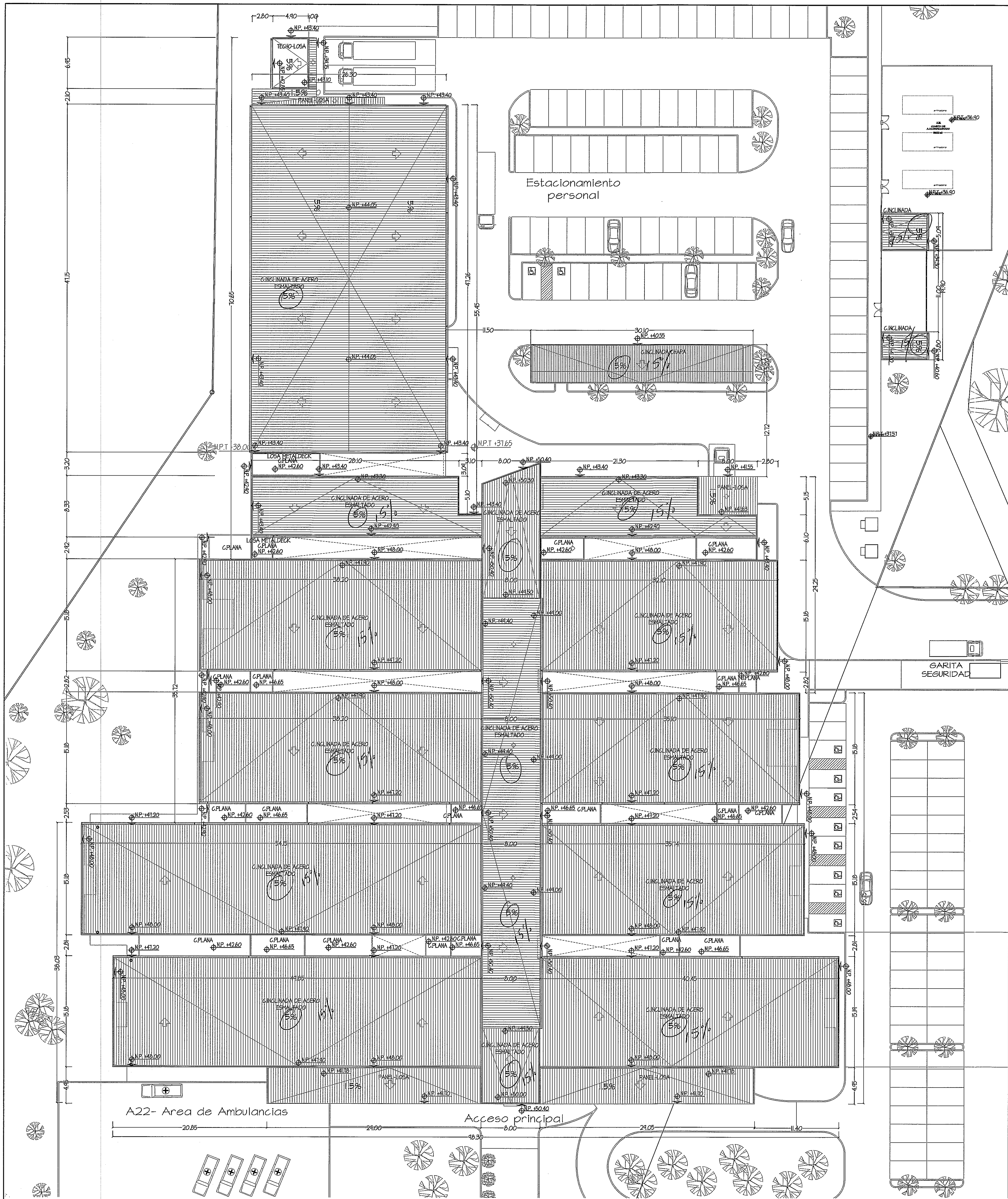
PLANTA DE TECHO ARQUITECTONICA (NIVEL 200) ESCALA.- 1/250
