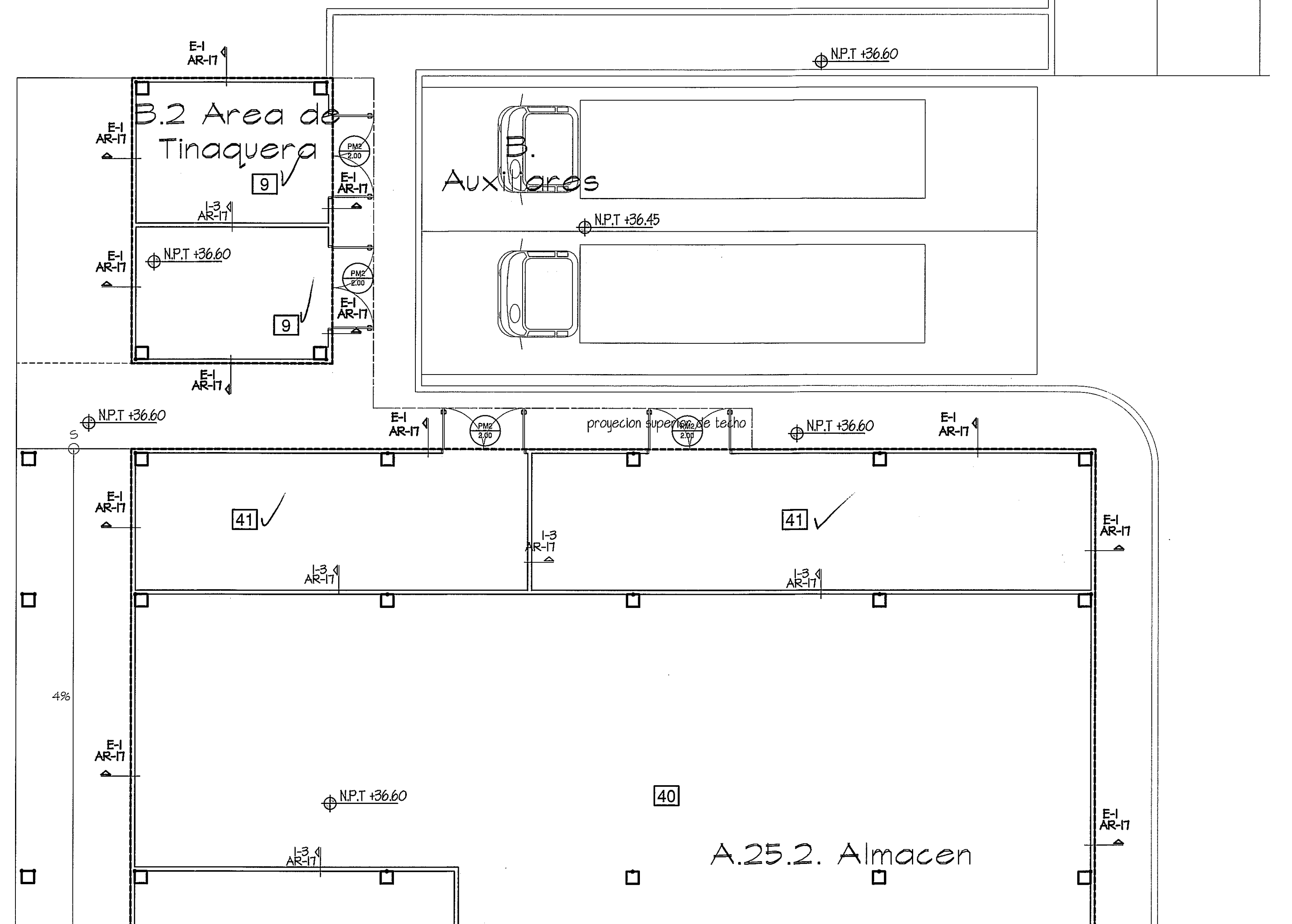
AMPLIACION DE ZONA 1/2 PLANTA BAJA ESCALA.- 1/75
