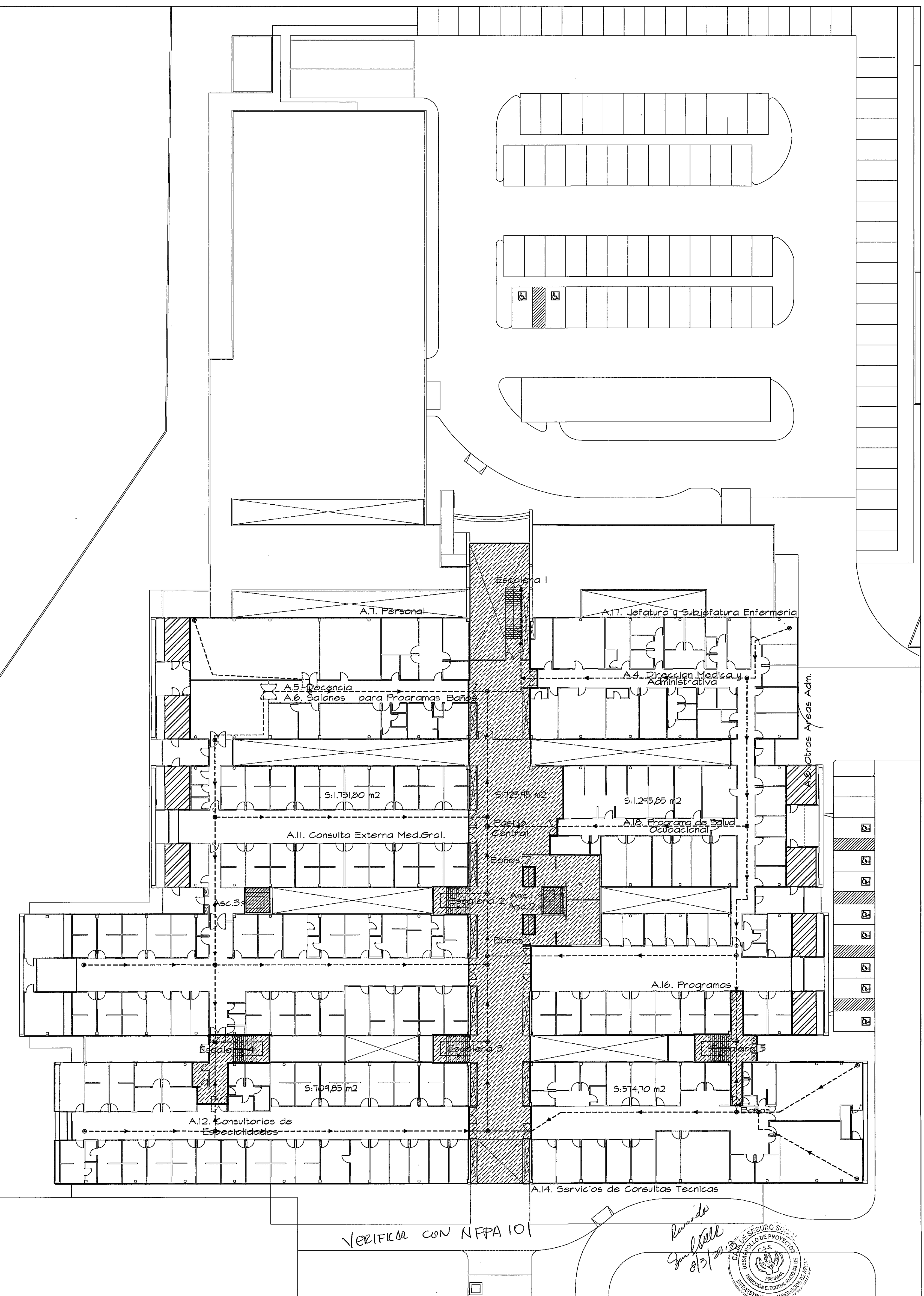
PLANTA ALTA ARQUITECTONICA NIVEL 100) ESCALA.- 1/250
