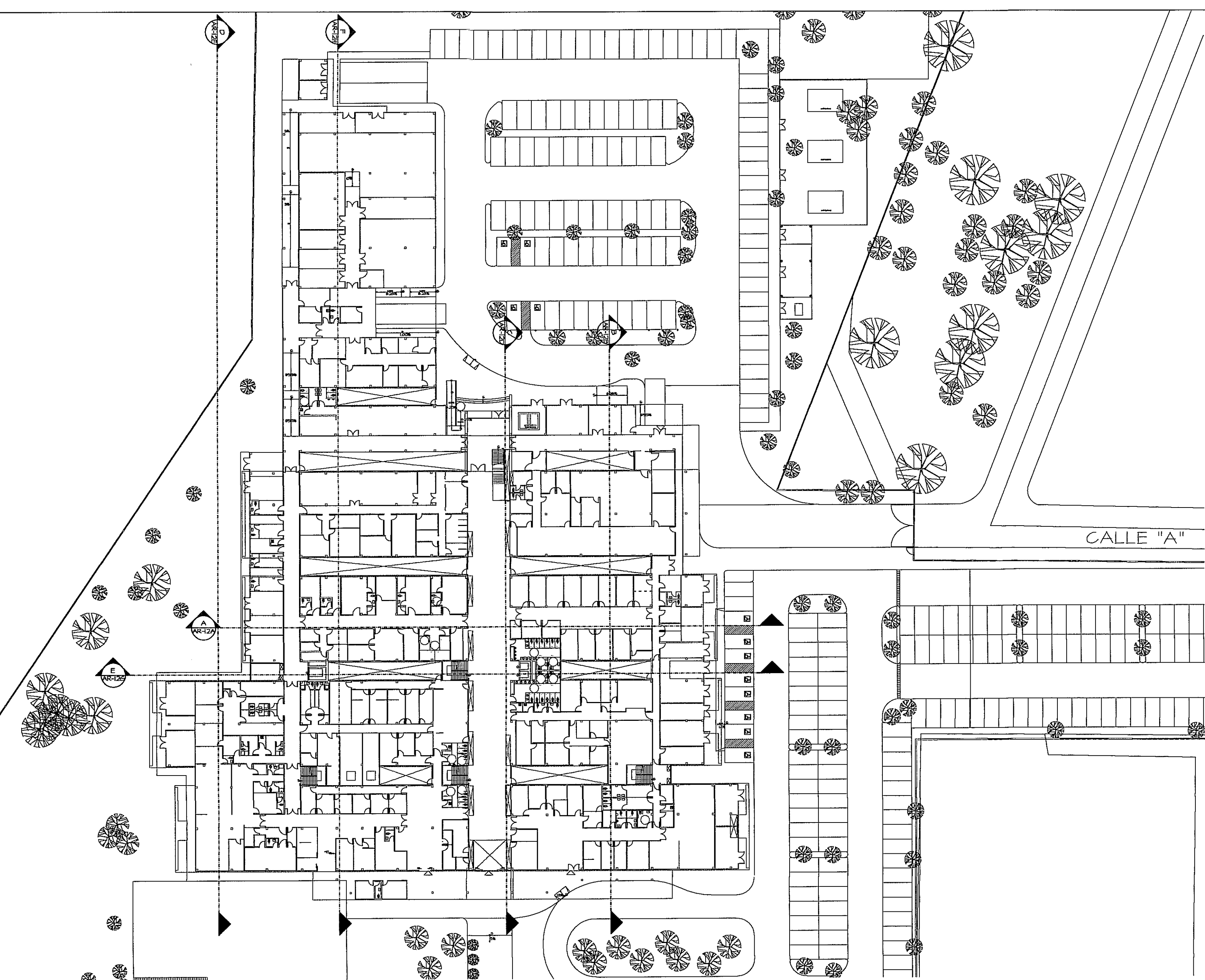
PLANTA BAJA ARQUITECTURA ESC. 1:500
