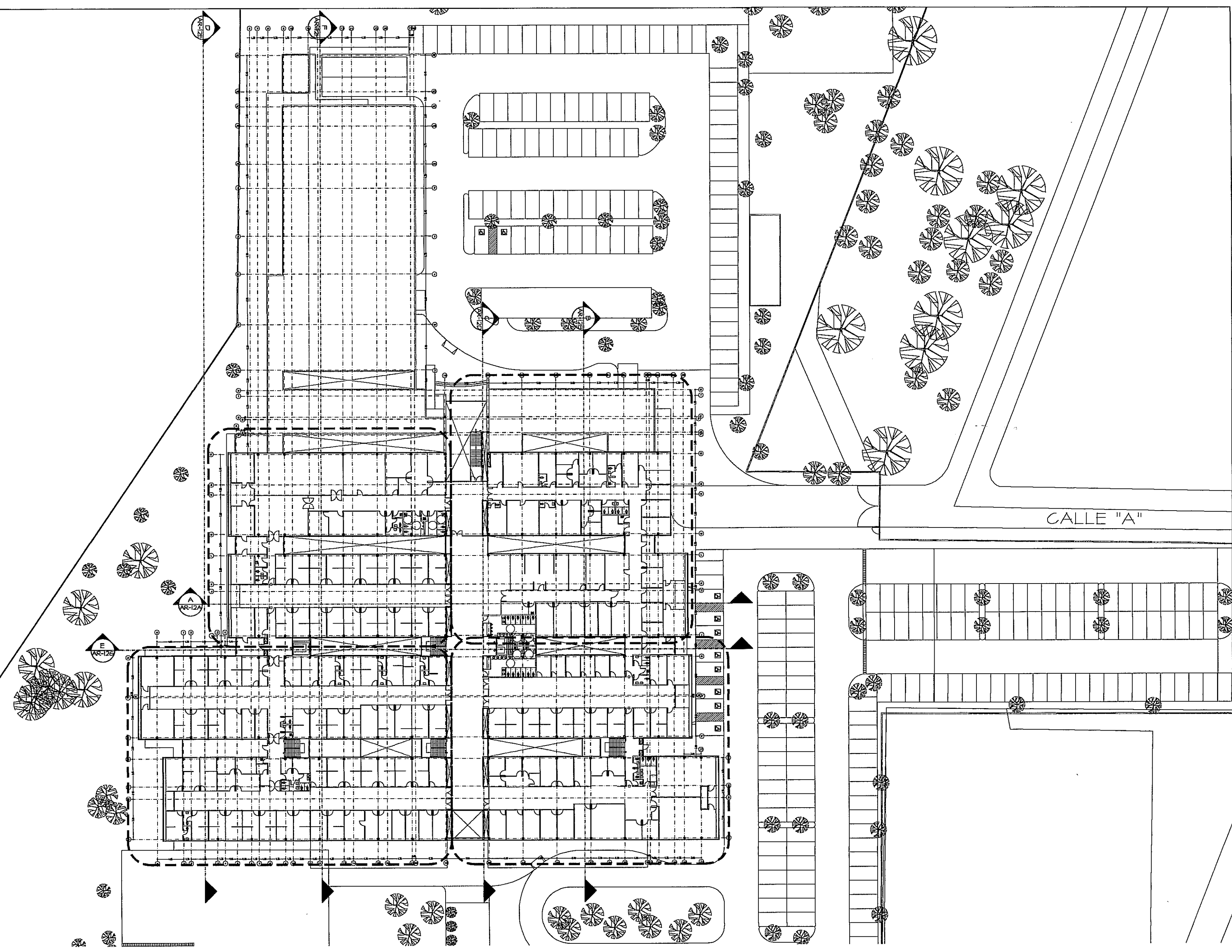
PLANTA ALTA ARQUITECTURA ESC. 1:500
