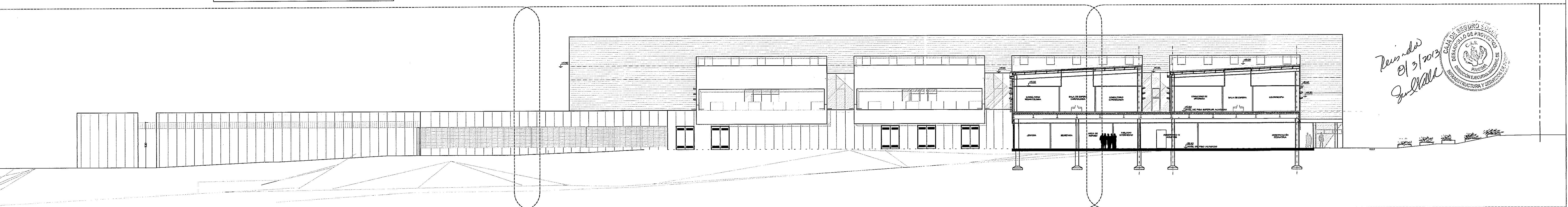
SECCION D-D ESC. 1:200
