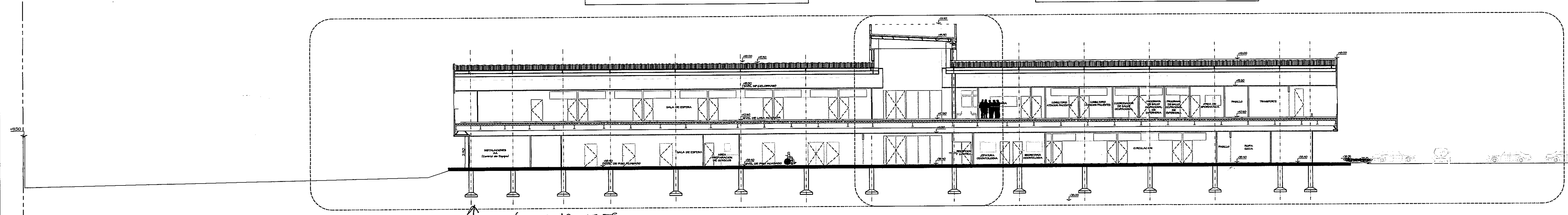
SECCION TRANSVERSAL ESC. 1:200
