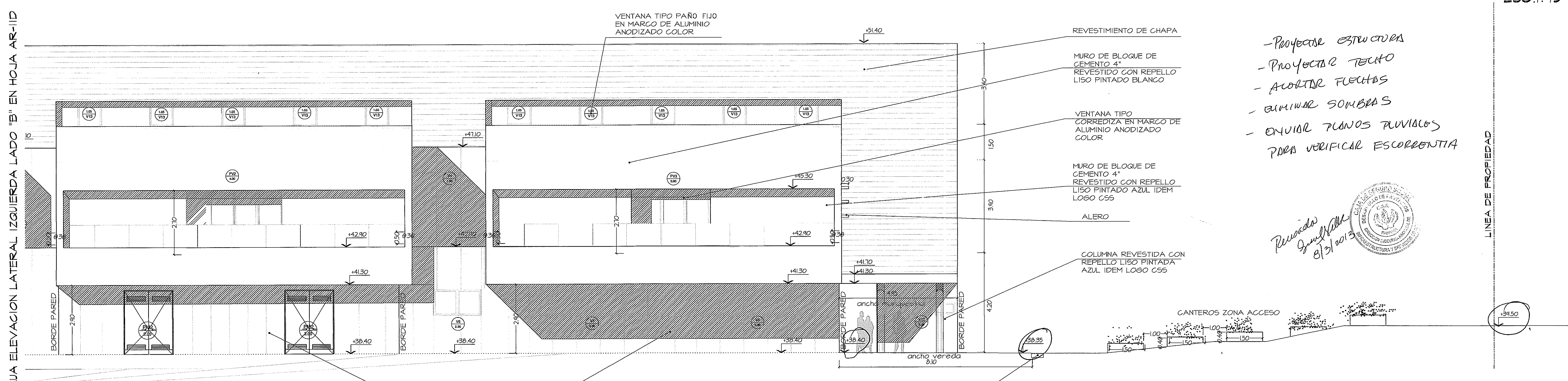
ELEVACION LATERAL IZQUIERDA - AMPLIACION LADO "C" ESC.1:75
