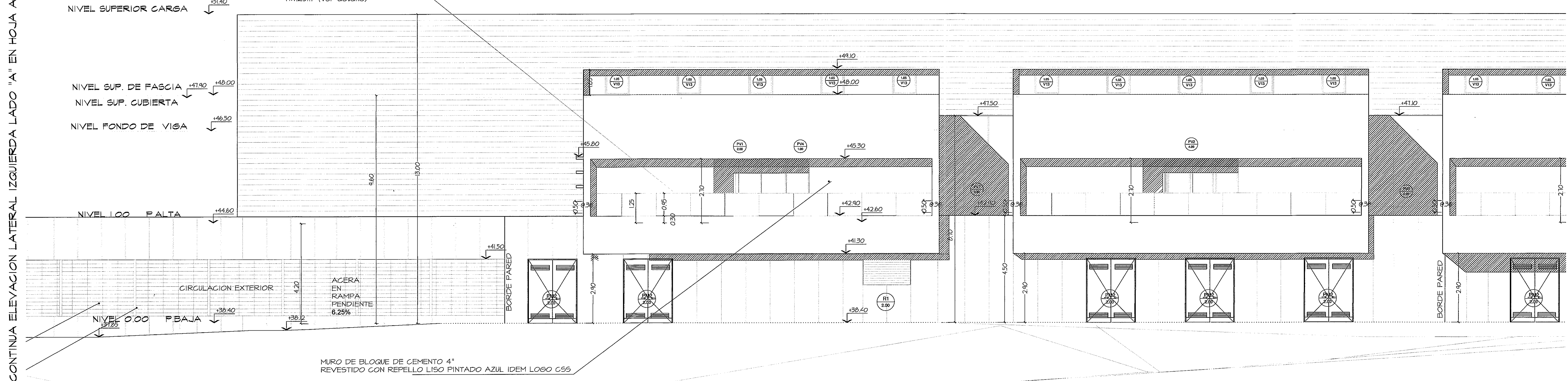
ELEVACION LATERAL IZQUIERDA - AMPLIACION LADO "B" ESC.1:75
