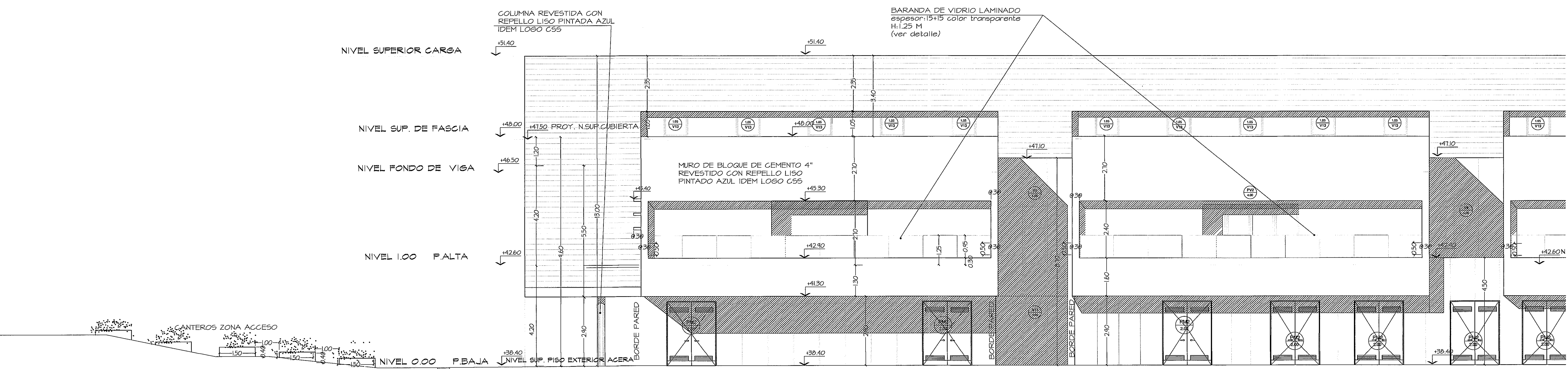
ELEVACION LATERAL DERECHA - AMPLIACION LADO "A" ESC. 1:75
