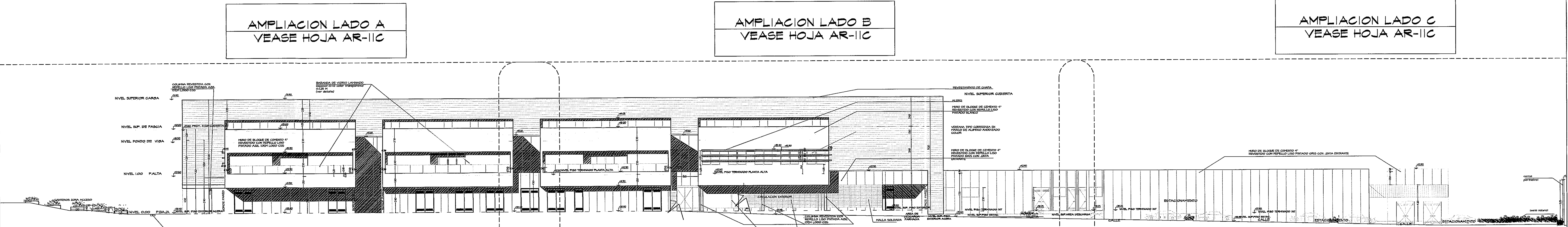
ELEVACION LATERAL DERECHA ESC. 1:200
