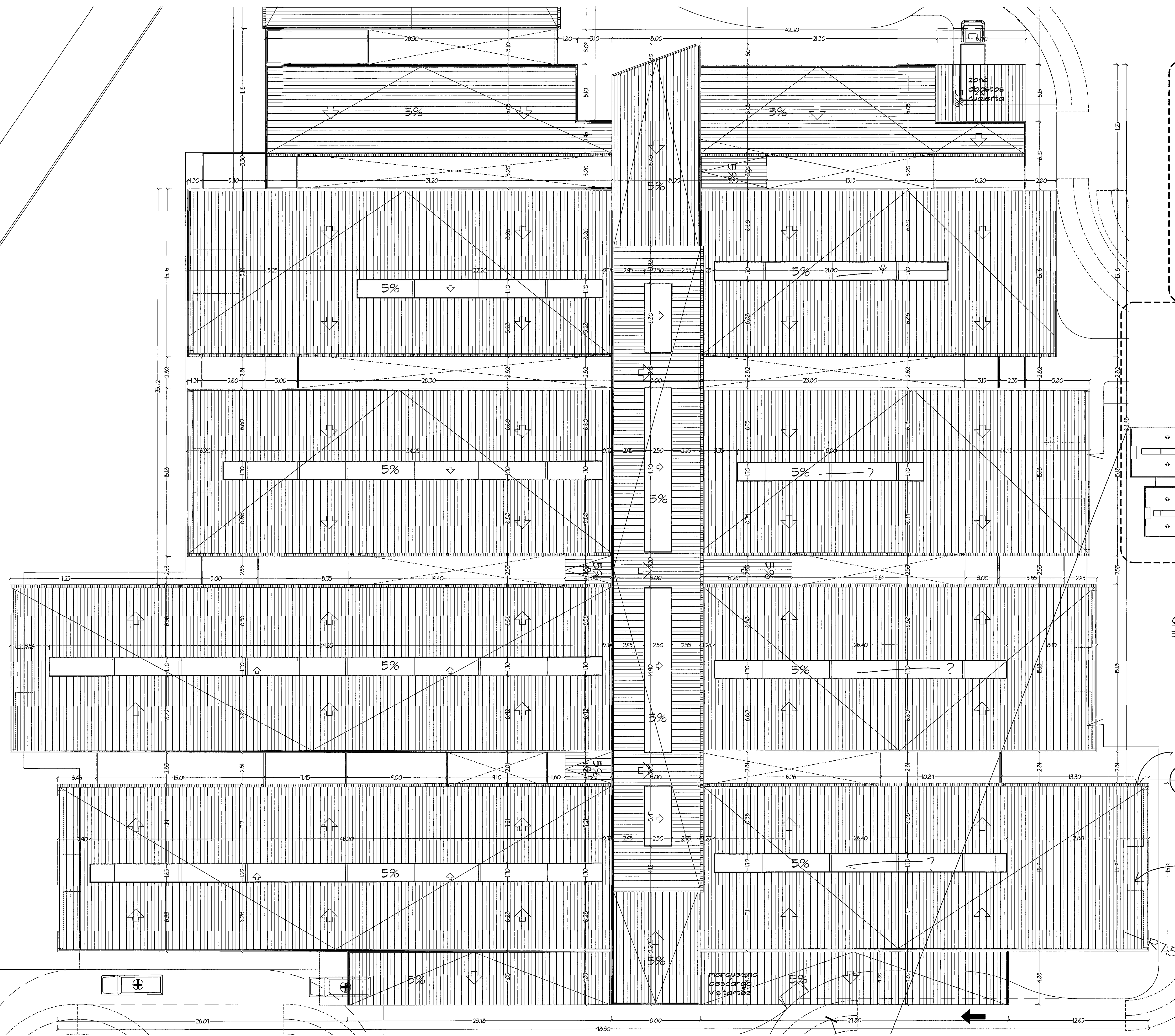
AMPLIACION DE ZONA 10 PLANTA DE TECHO ESCALA.- 1/150
