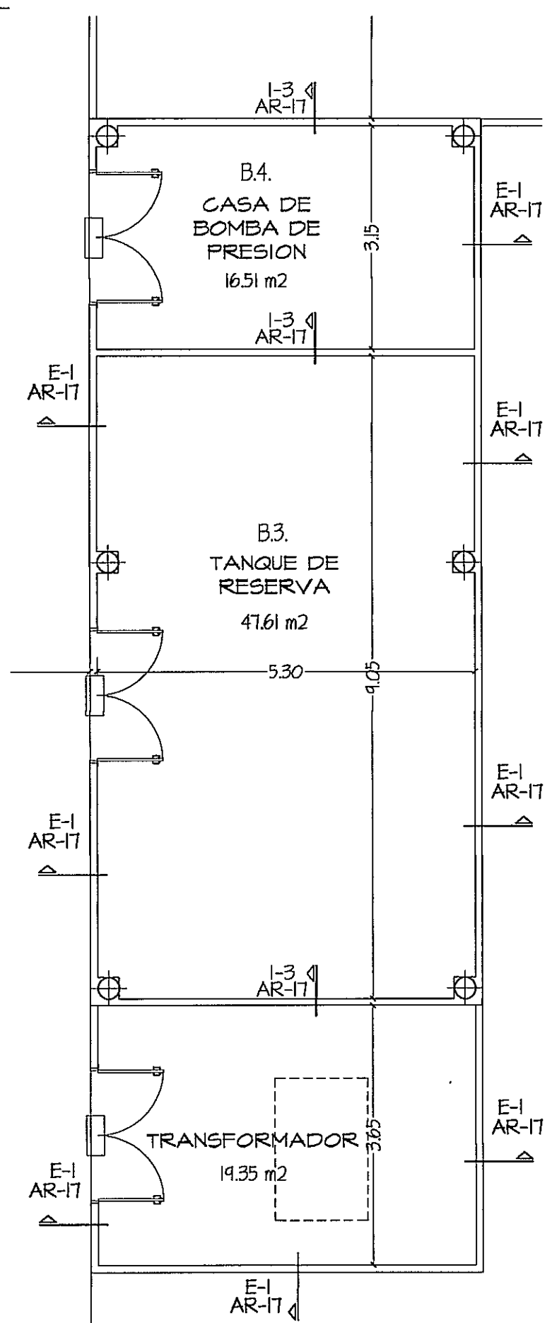
AMPLIACION DE ZONA 4/2 PLANTA BAJA ESCALA.- 1/75
