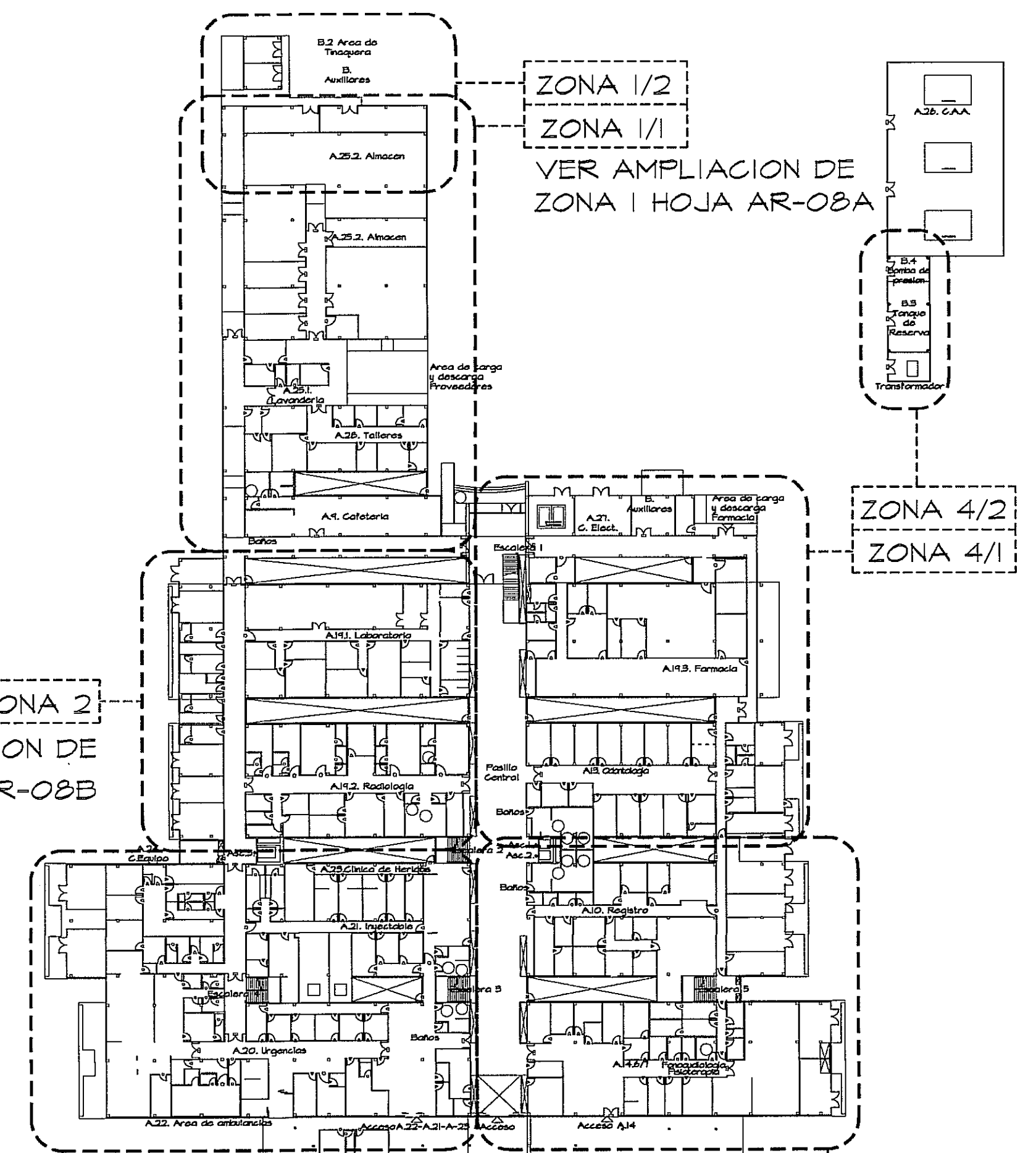
VER AMPLIACION DE ZONA 3 HOJA AR-08C VER AMPLIACION DE ZONA 5 HOJA AR-08E
