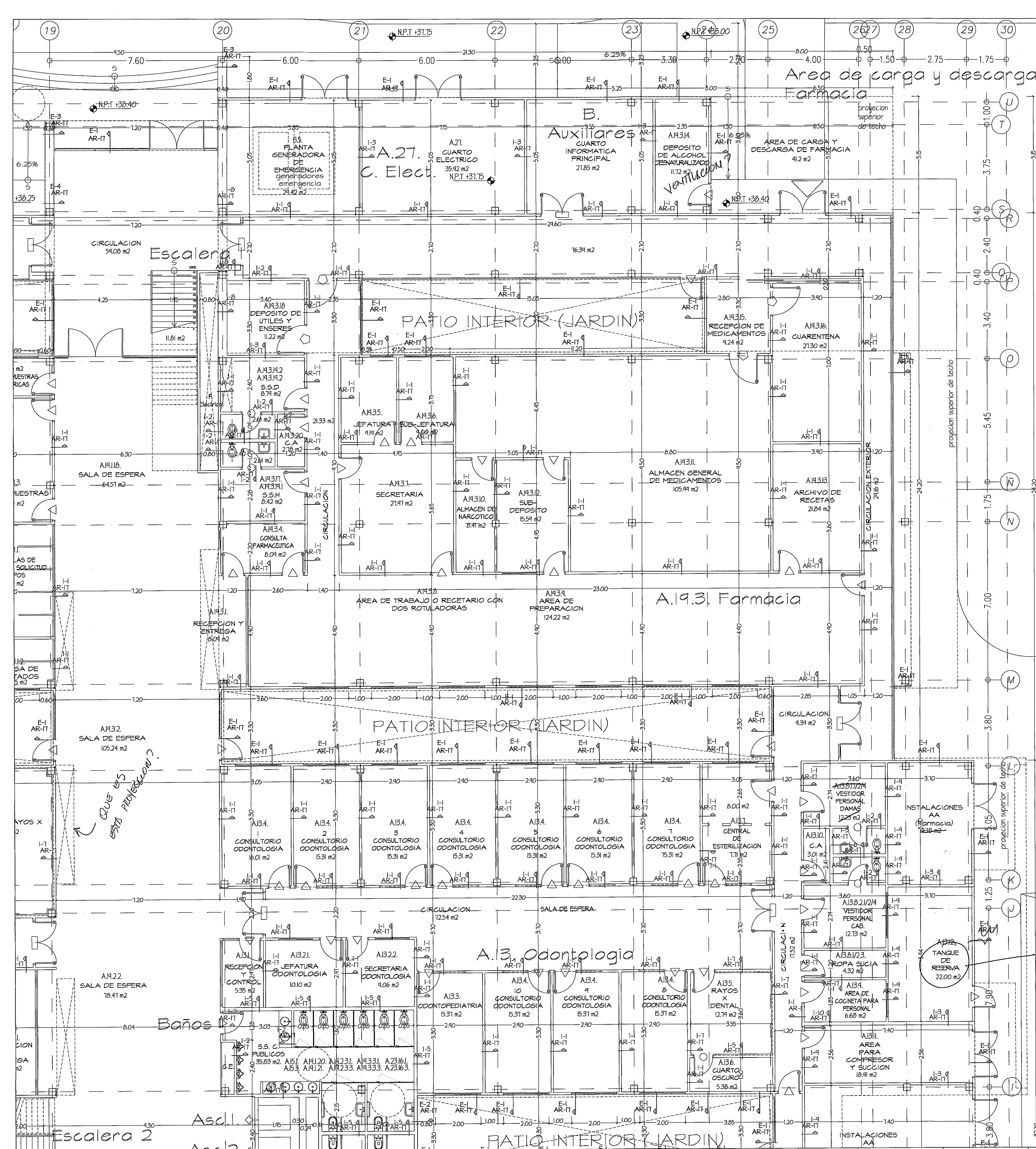
VER AMPLIACION DE ZONA 2 HOJA AR-08B
