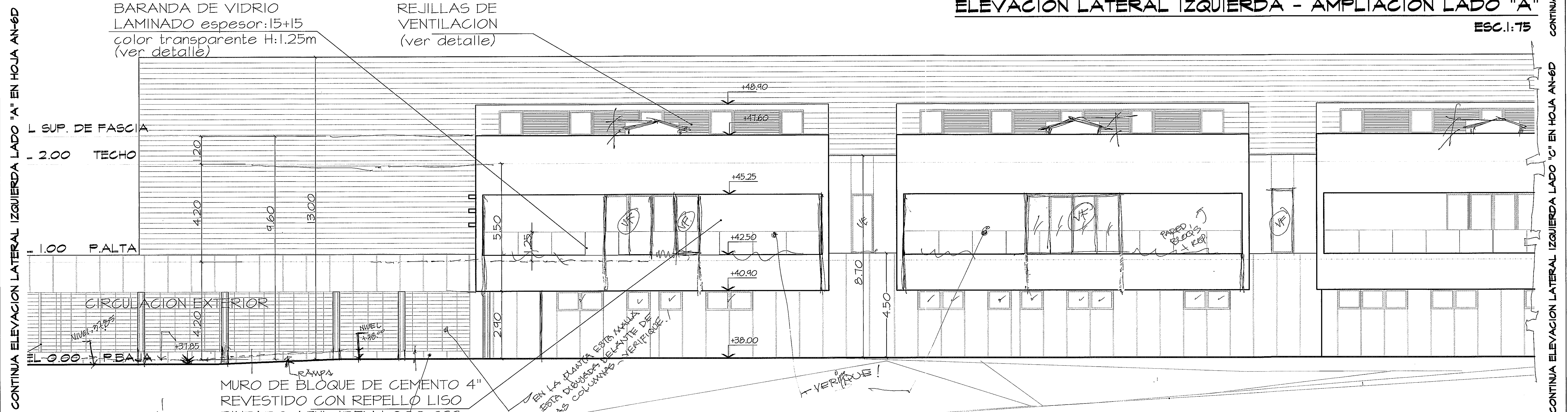
ELEVACION LATERAL IZQUIERDA - AMPLIACION LADO "B" ESC.1:75
