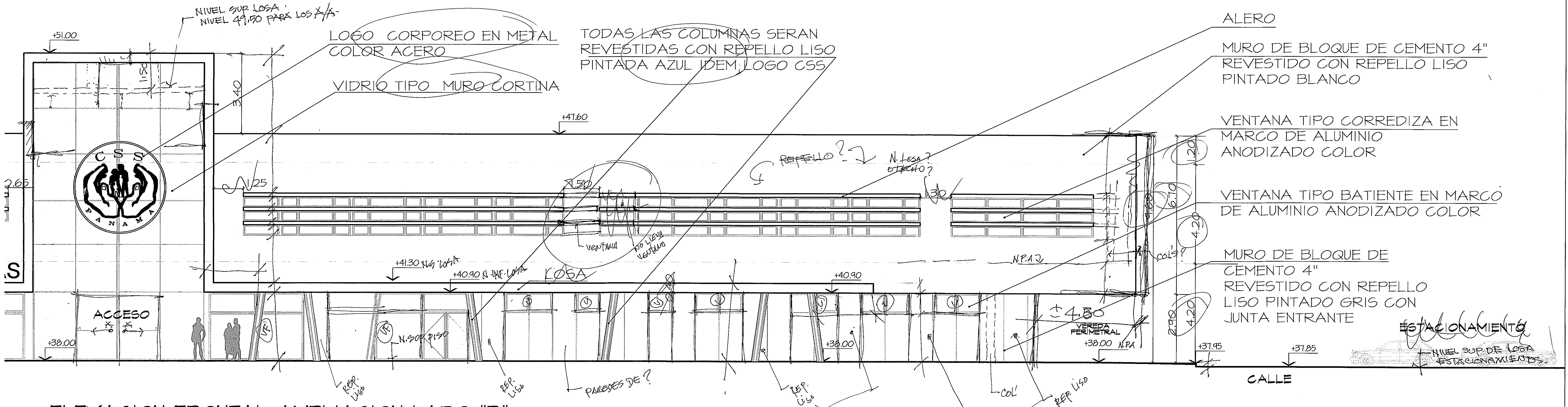
ELEVACION FRONTAL-AMPLIACION LADO "B" ESC.1:75
