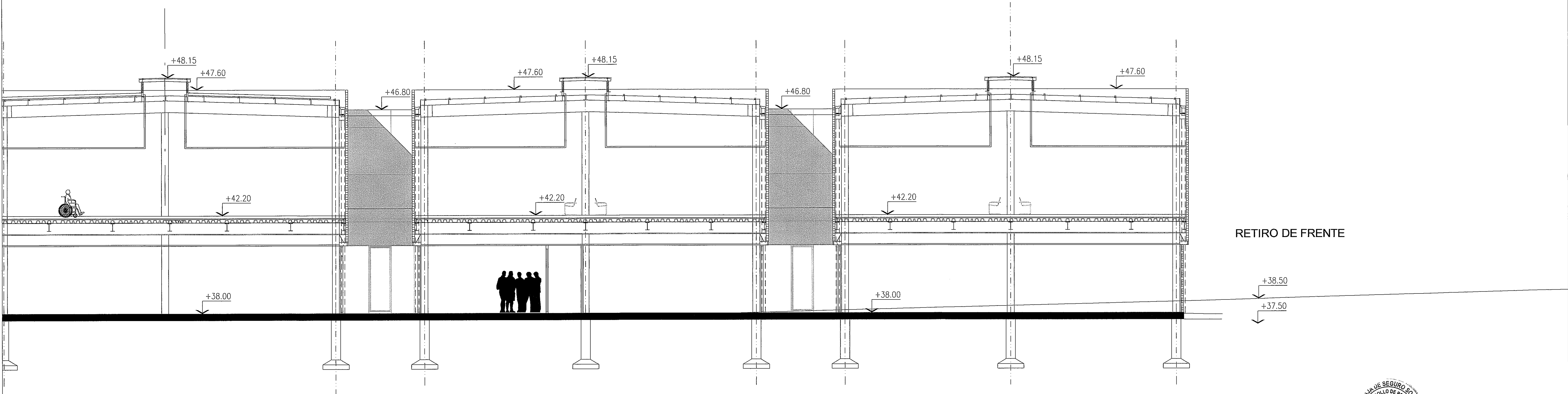
CORTE B-B
